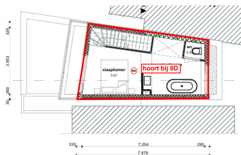
2E VERDIEPING
