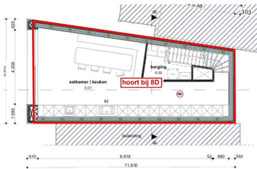
SOUTTERAIN
