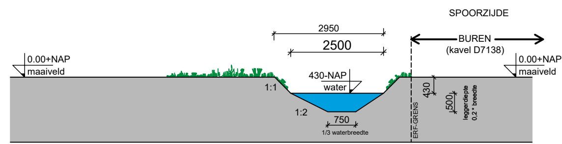
secundair boezemwater - doorsnede W1 Bestaand 1:100
