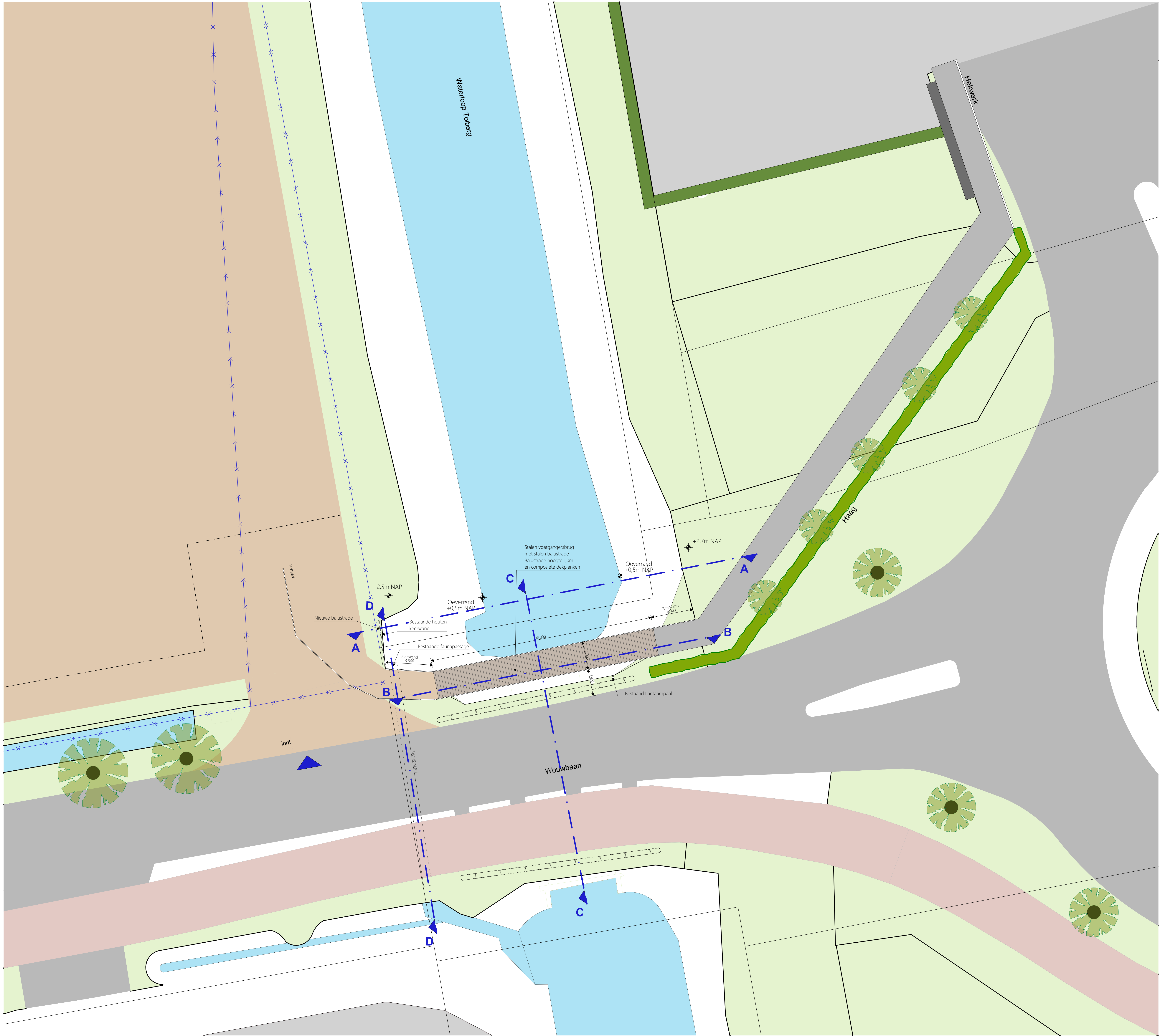
Terreinplan nieuw - stalen brug 1:100
