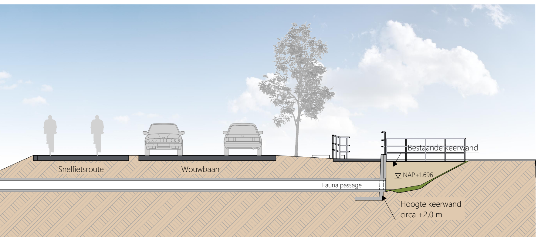
Doorsnede D - 1:100
