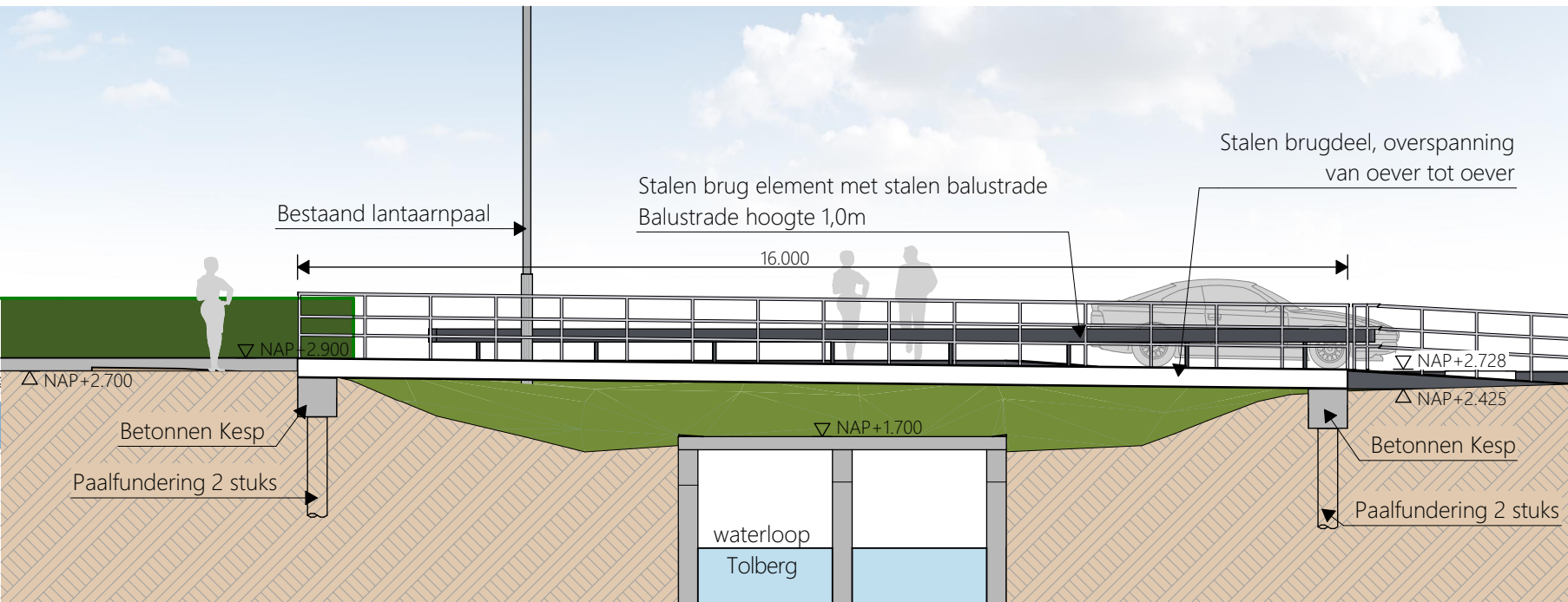
Doorsnede B - 1:100
