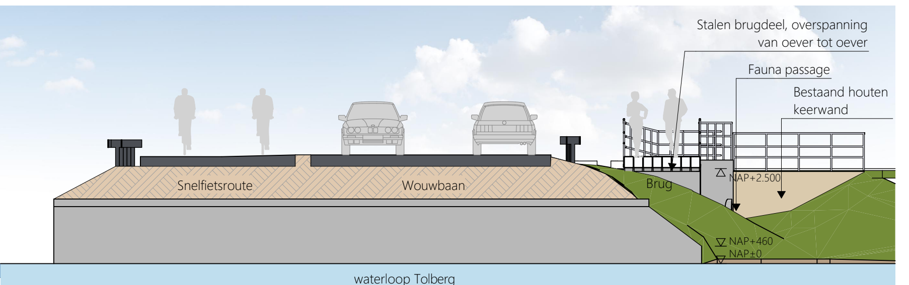
Doorsnede C - 1:100
