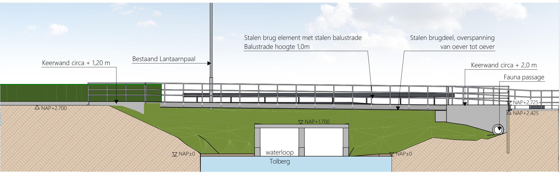
Doorsnede A - 1:100
