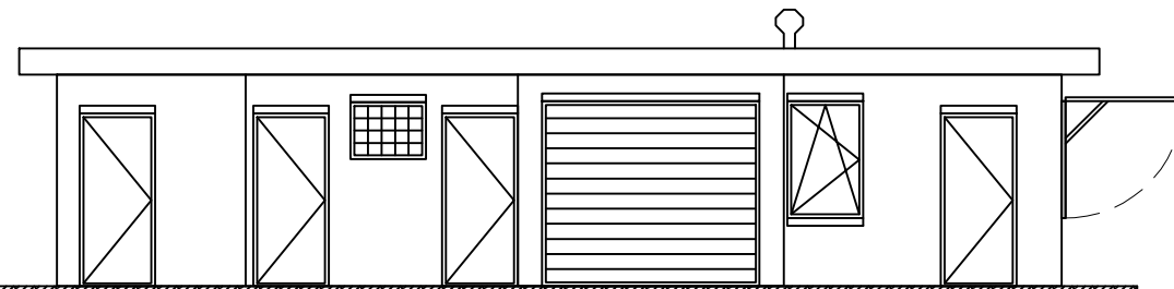
oostgevel (gewijzigd)
