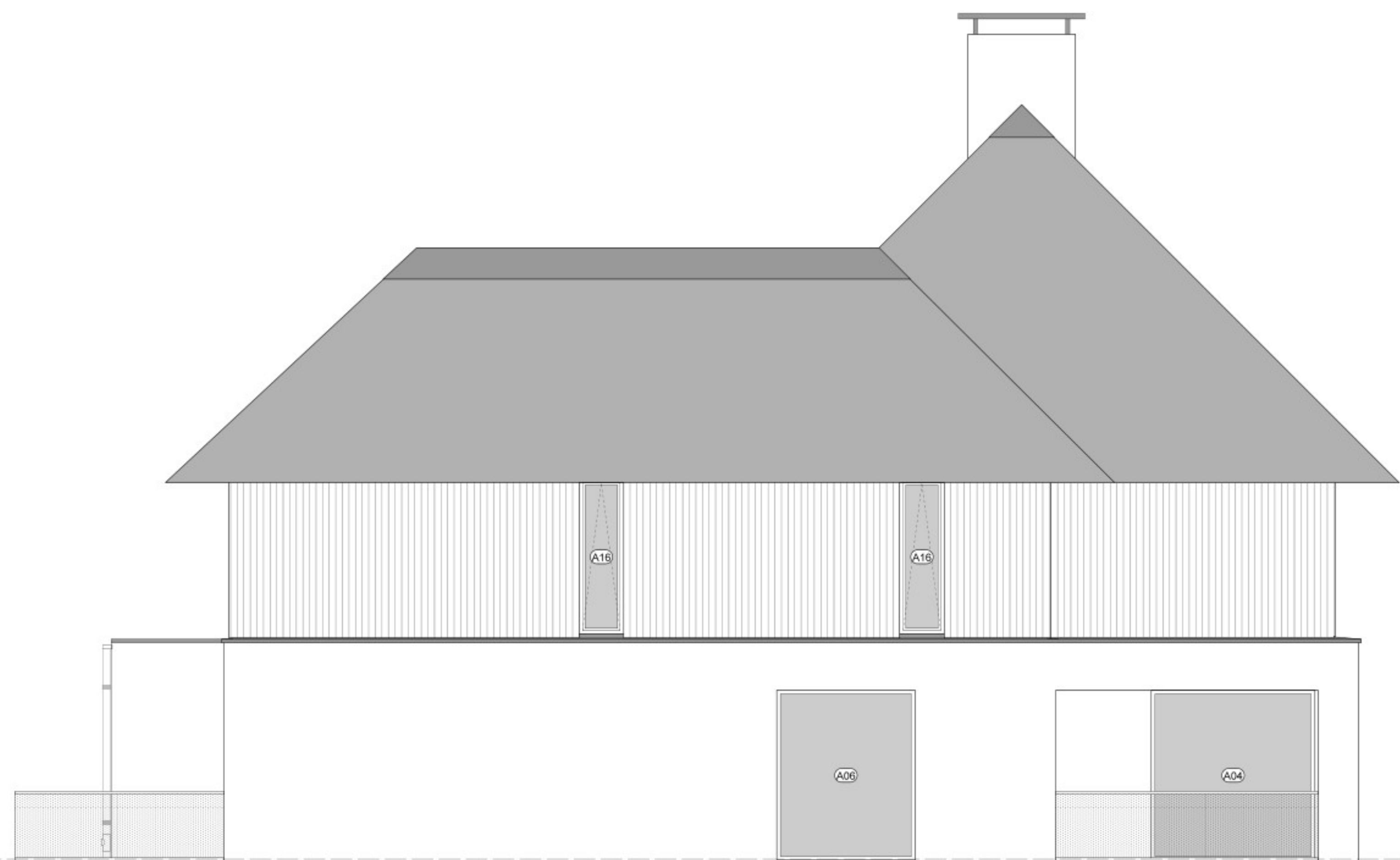
Gevel links
