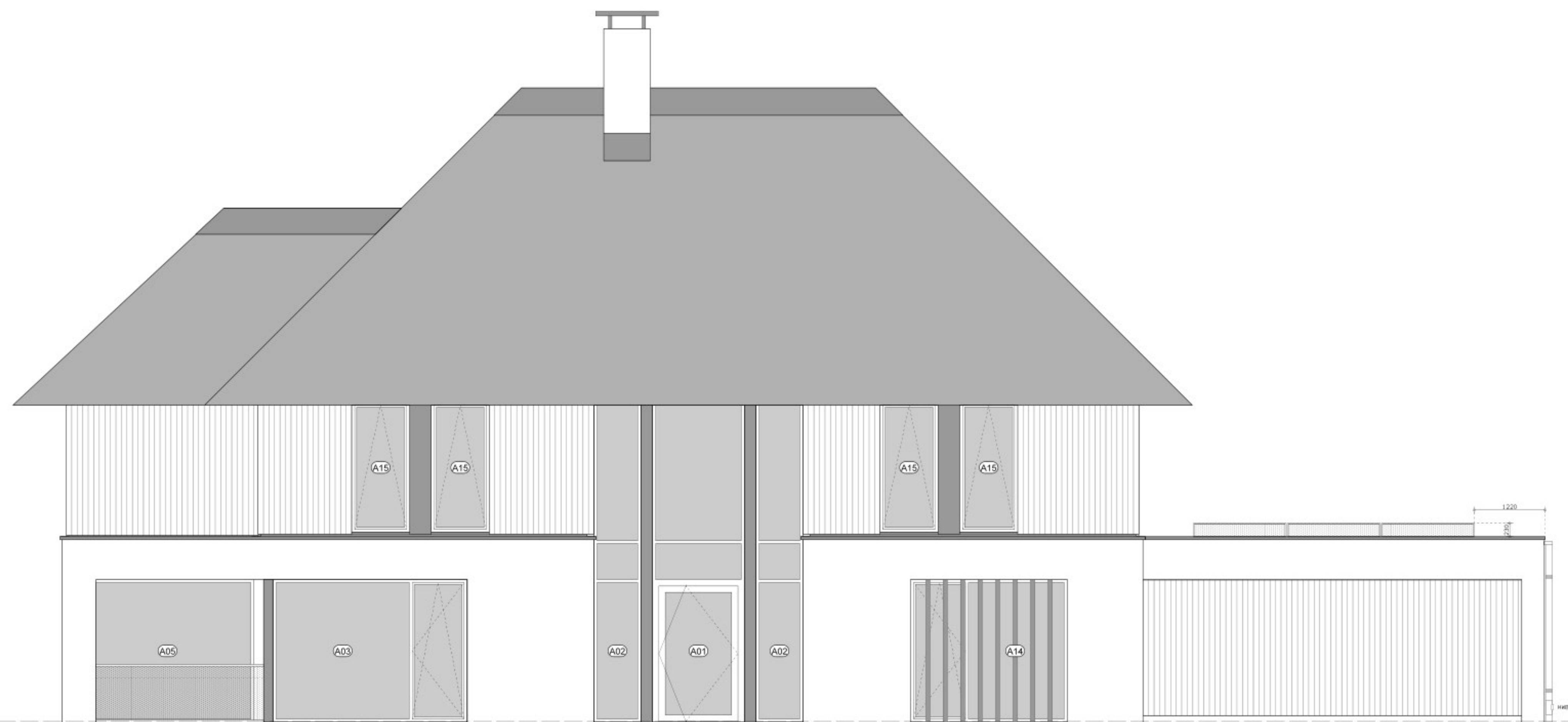
Voorgevel
