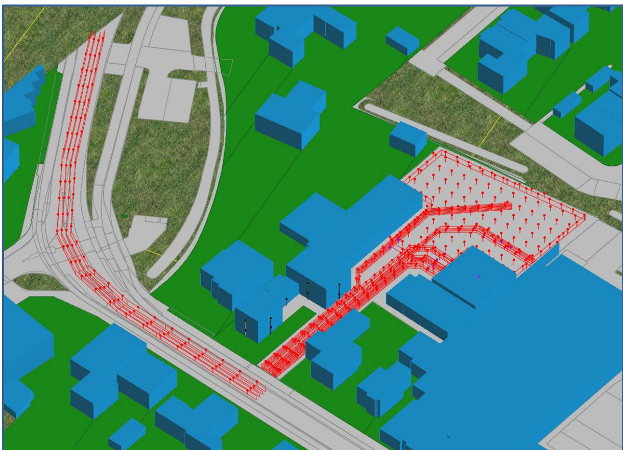
Afbeelding 4. Rekenmodel, 3d-weergave
