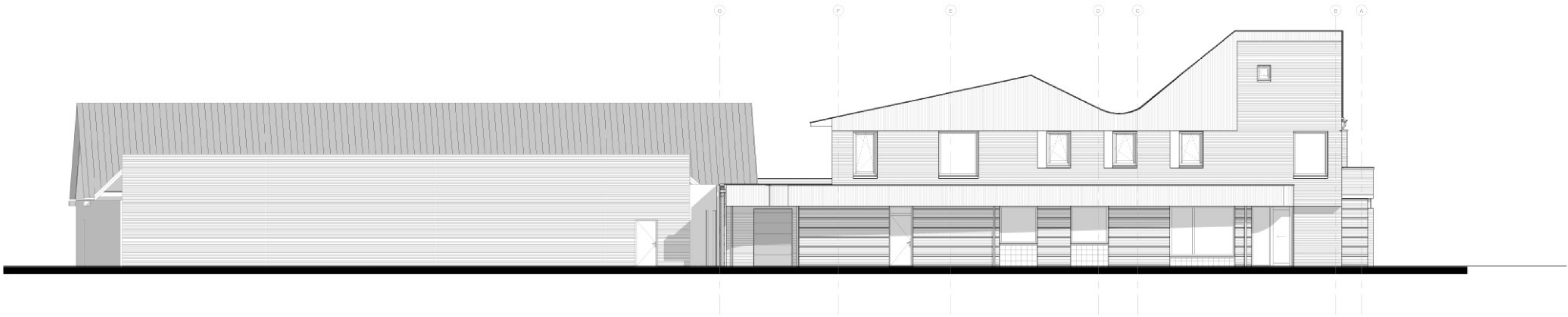
Linker zijgevel
