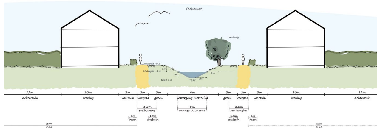
Figuur 23: Dwarsprofiel landschapslijnen met polderidentiteit
