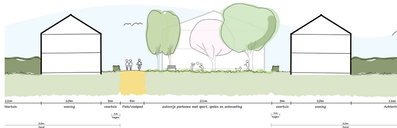
Figuur 26: Dwarsprofiel parkachtige dwarsverbindingen
