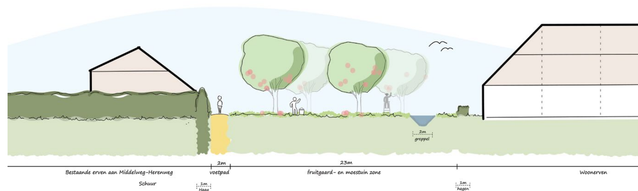
Figuur 27: Dwarsprofiel landelijke groenbuffer achter polderlint
