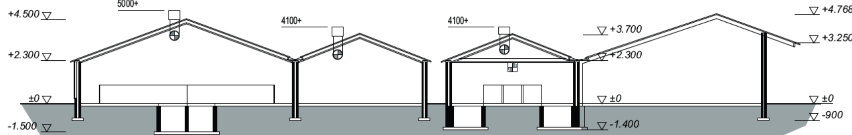
Doorsnede C - C
