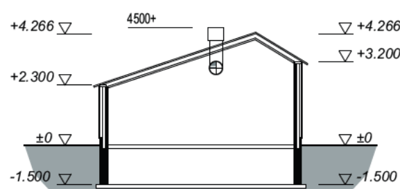
Doorsnede D - D
