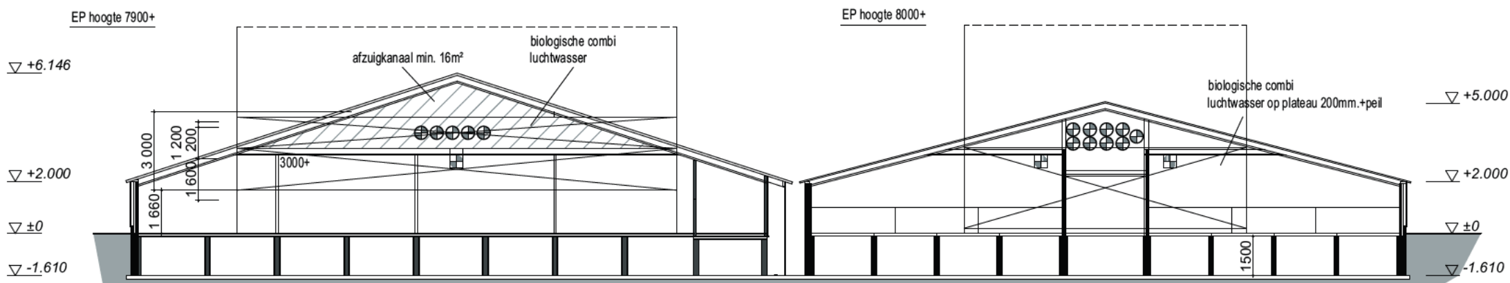
Doorsnede A - A
