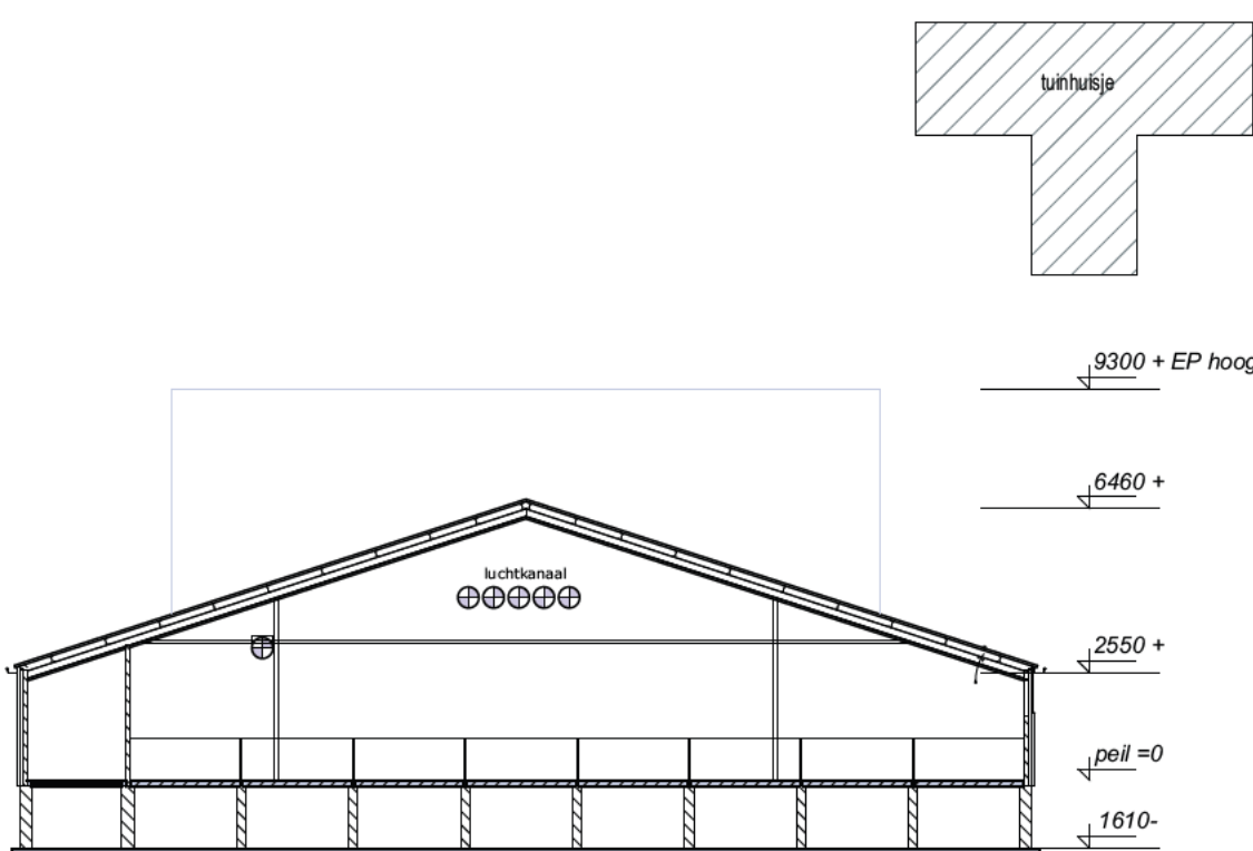
doorsnede B-B
