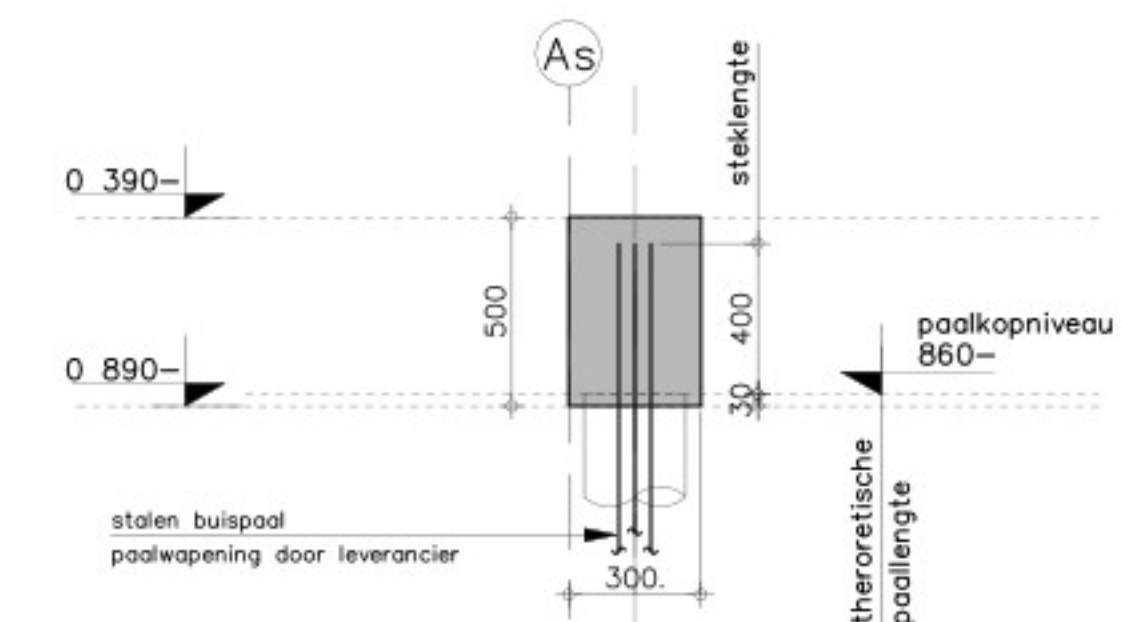
Algemeen paalkopdetail 1:20
