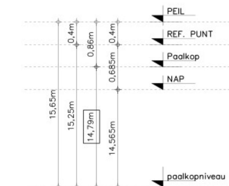
Paallengte 1:20
