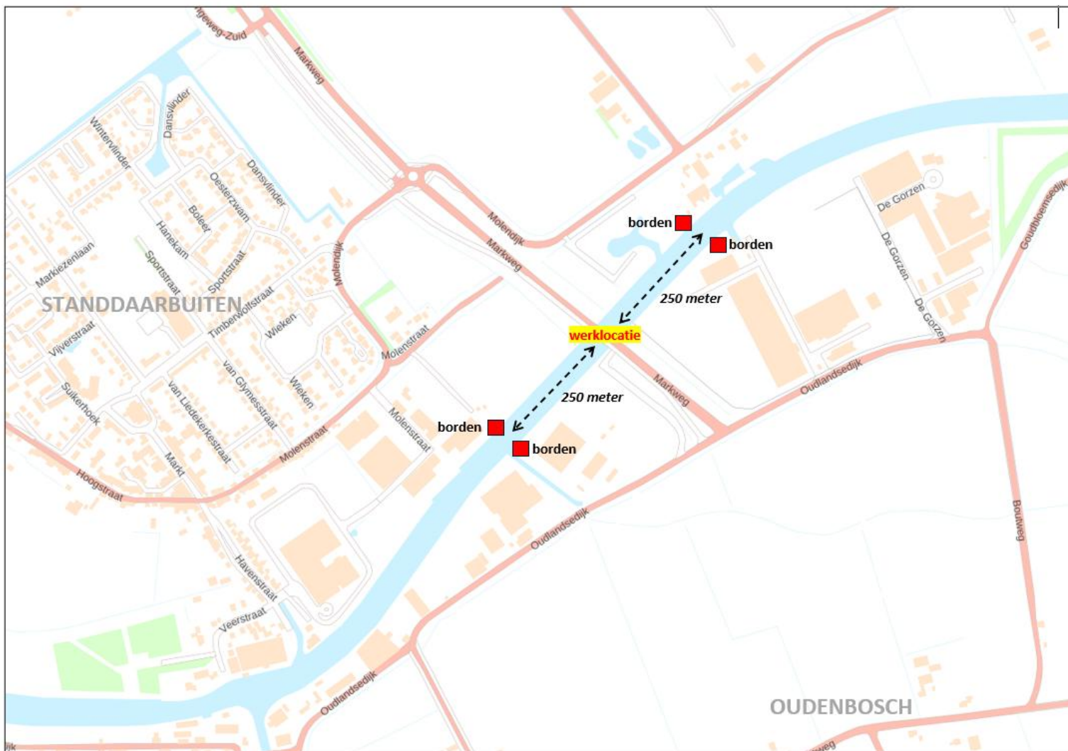
Scheepvaartbord B.8
