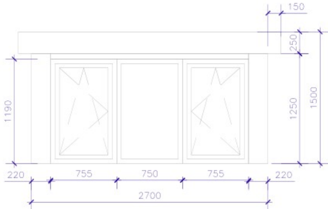
Aanzicht dakkapel voorgevel 1:25
