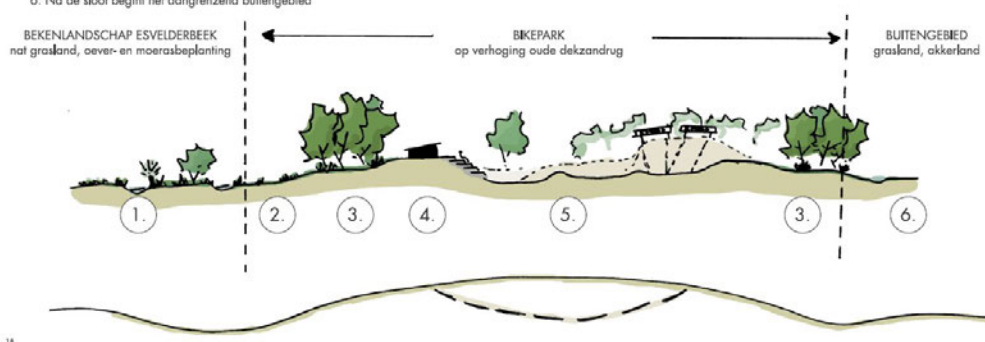
Figuur 4 Doorsnede van het plangebied. Tussen de BMX baan en de bomenrij aan het zuiden van het plangebied loopt een weg die 2,5 meter hoger ligt dan de BMX baan en de bomenrij.
