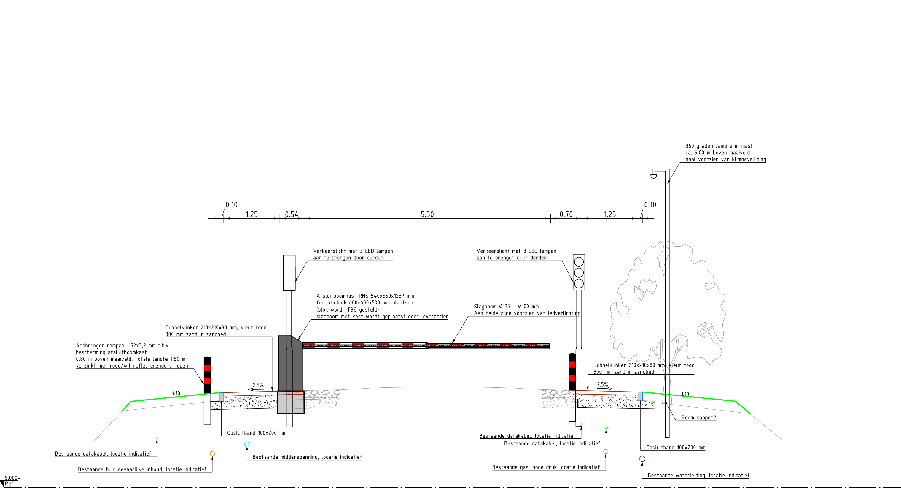
Dwarsprofiel t.p.v. situatie 02 SCHAAL 1 : 50
