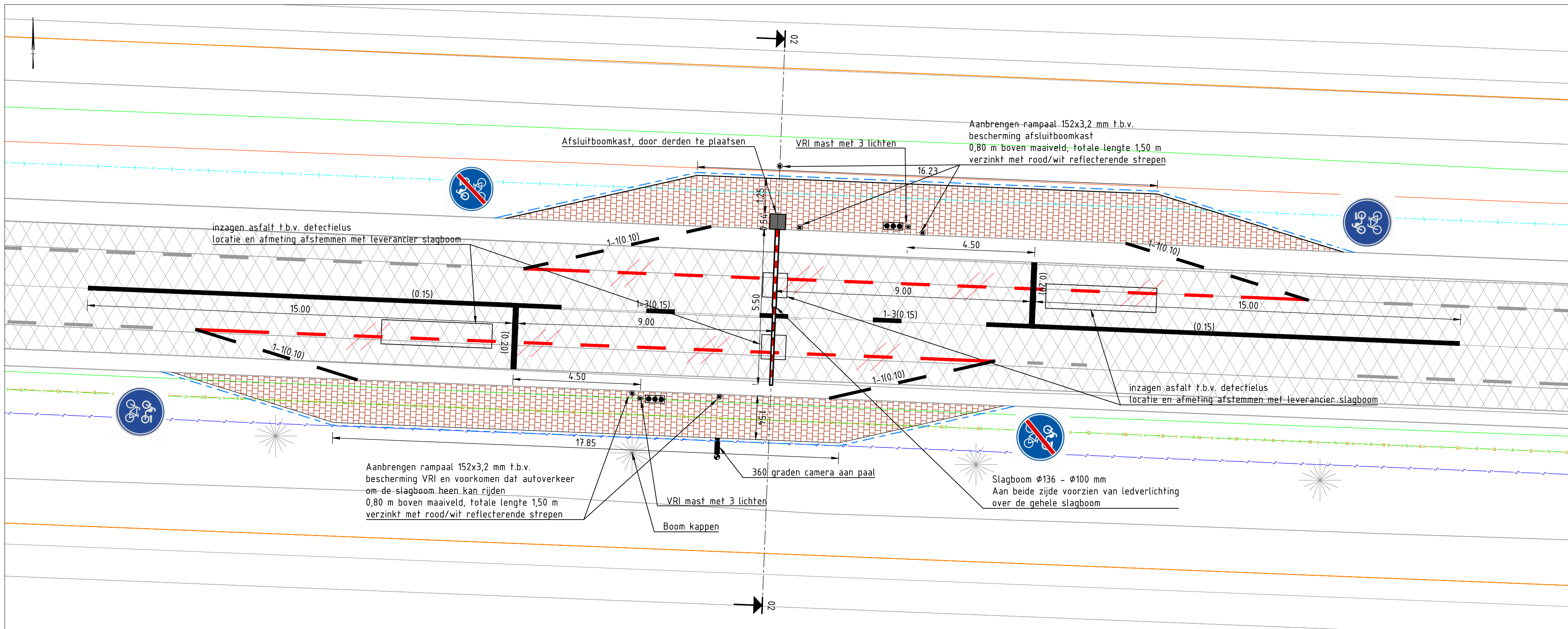
Situatie 02 "Slagboom locatie 02" SCHAAL 1 : 100
