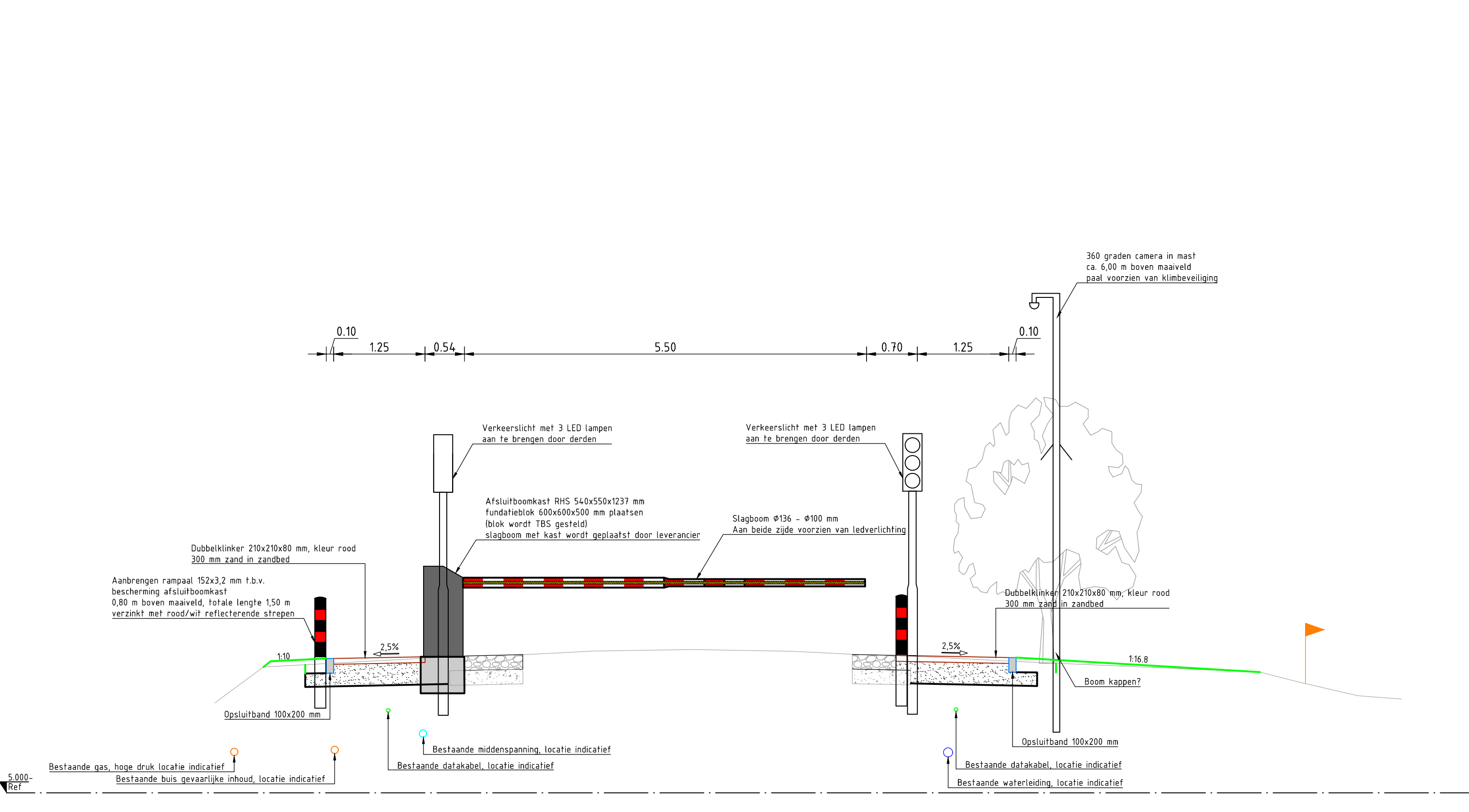
Dwarsprofiel t.p.v. situatie 01 SCHAAL 1 : 50
