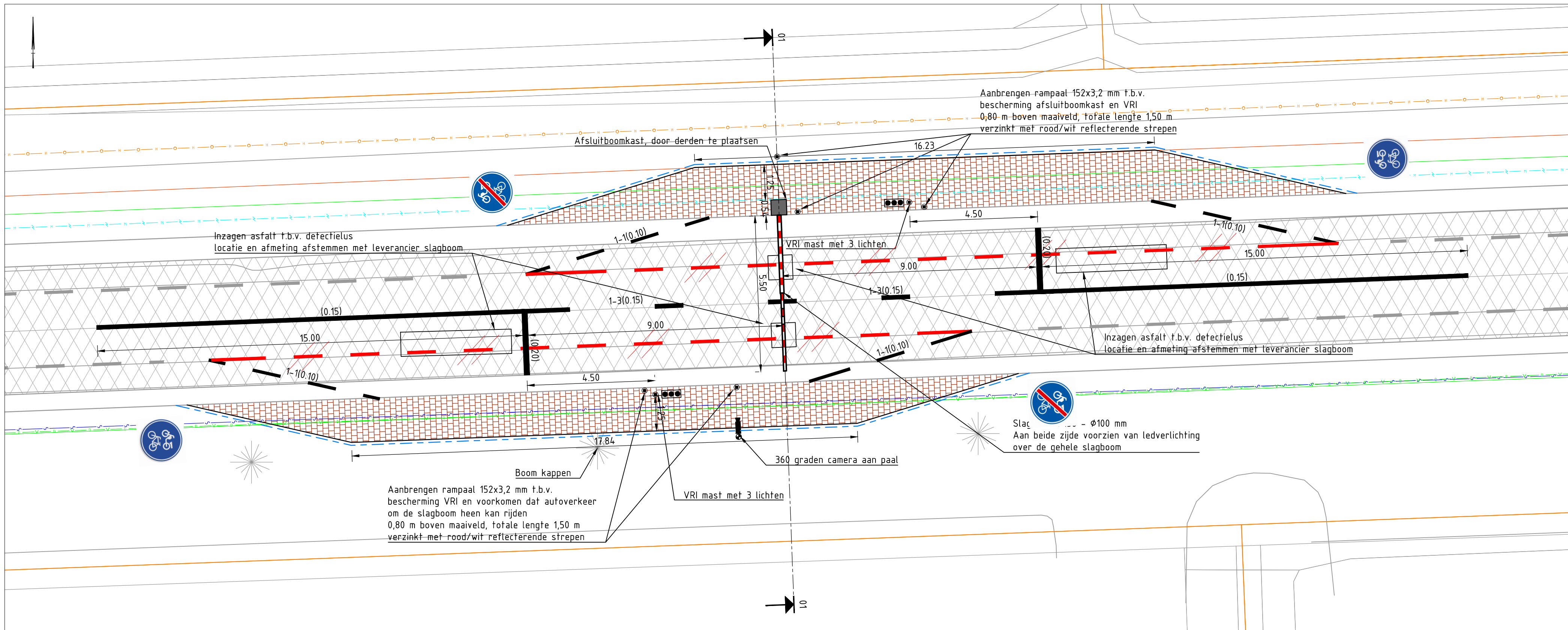
Situatie 01 "Slagboom locatie 01" SCHAAL 1 : 100
