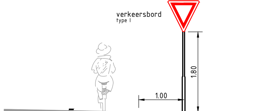
Principedetail bebording fietspad
