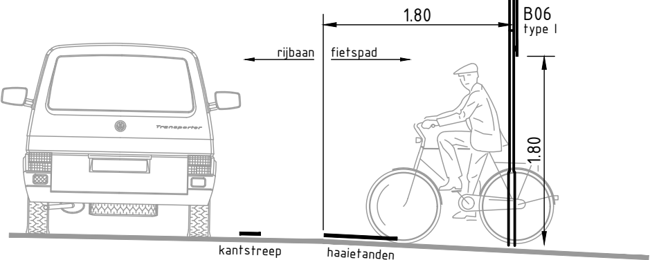
Principedetail bebording fietsoversteek
