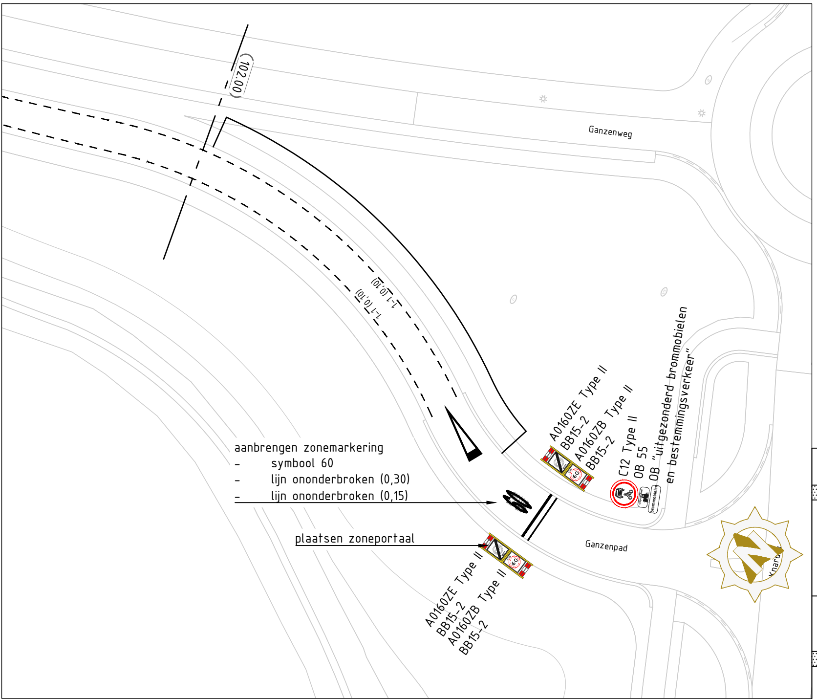
Situatie deel I km 101.98 – km 102.07
