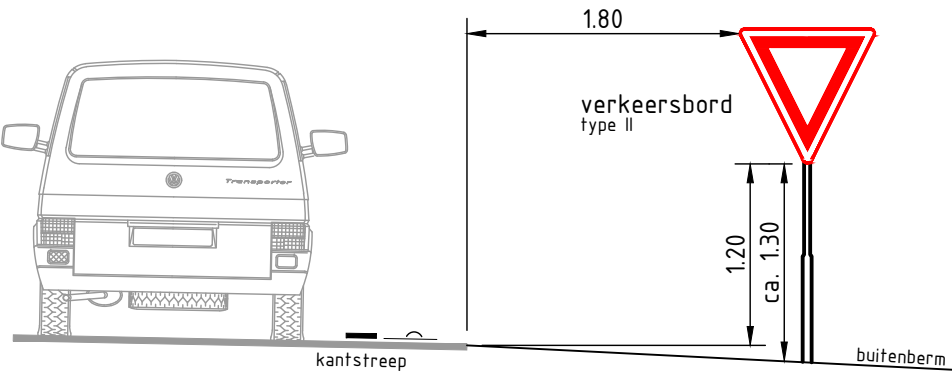
Principedetail bebording GOW en RSW
