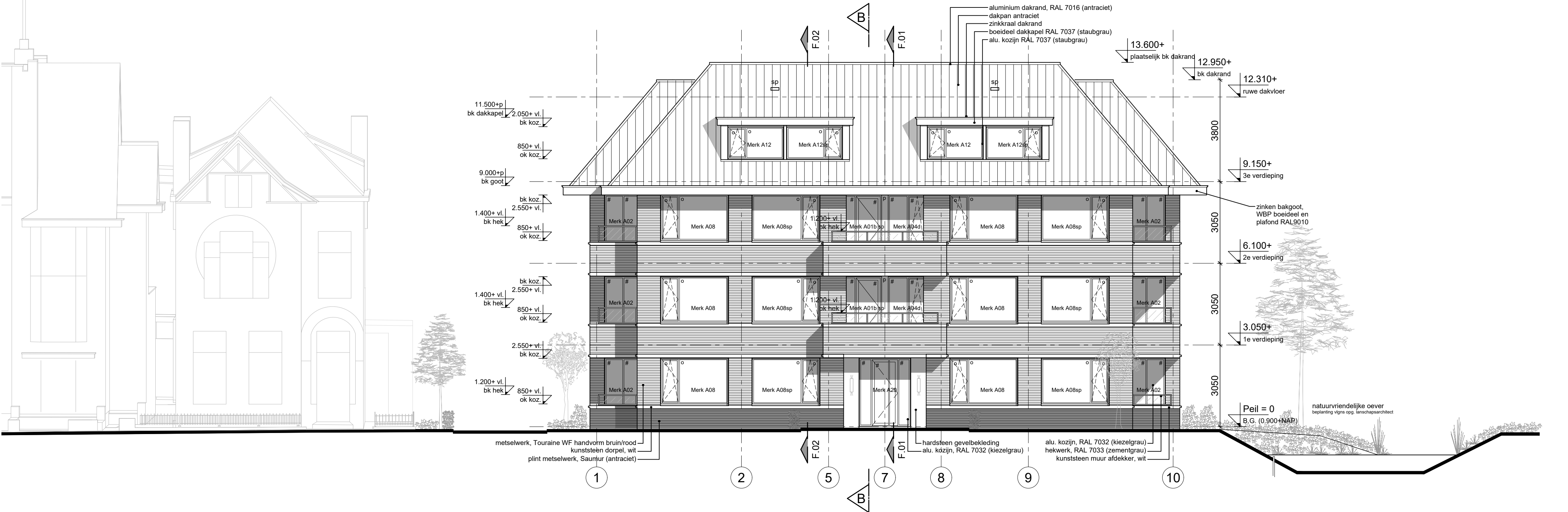
Voorgevel Zuidoost
