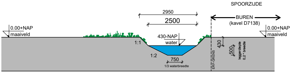
secundair boezemwater - doorsnede W1 Bestaand 1:100
