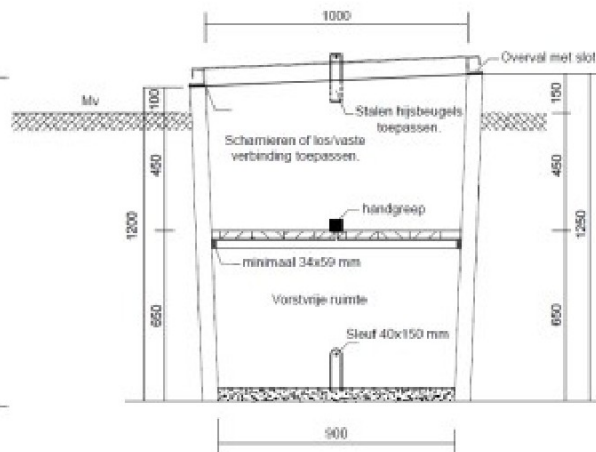
DOORSNEDE B - B
