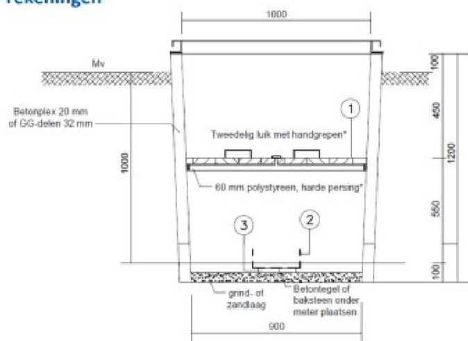
DOORSNEDE A - A
