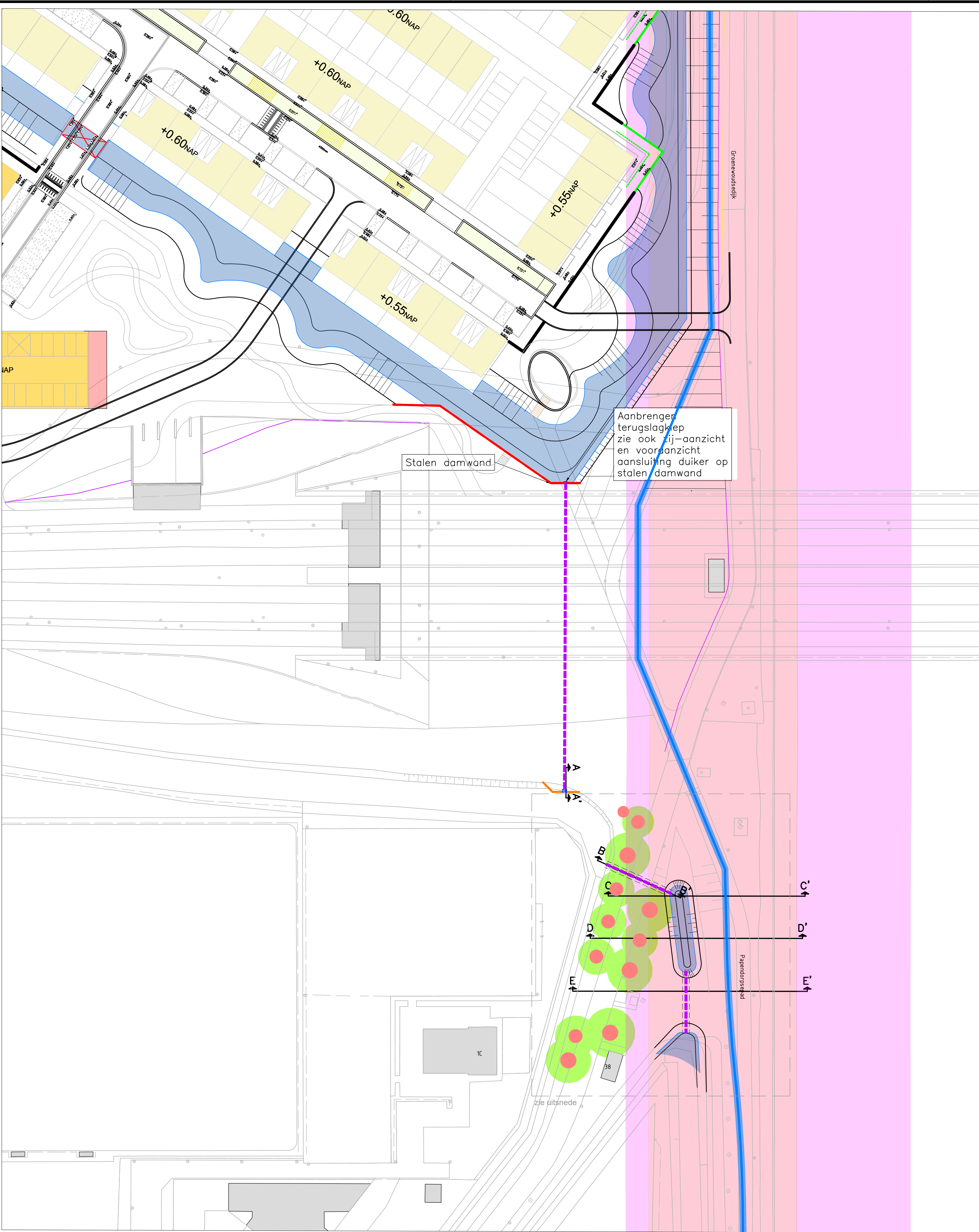
OVERZICHT schaal 1:500
