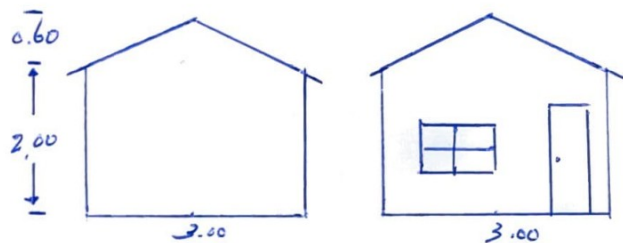
aanzicht kop
