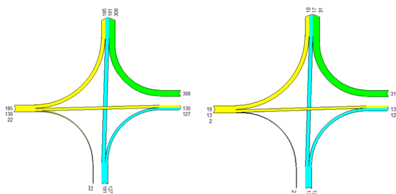
Figuur 5.3: Intensiteiten autoverkeer en vrachtautoverkeer planvariant (drukste ochtendspitsuur)
