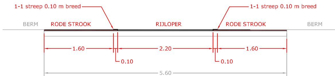
PRINCIPE PROFIEL 2 SCHAAL 1:50
