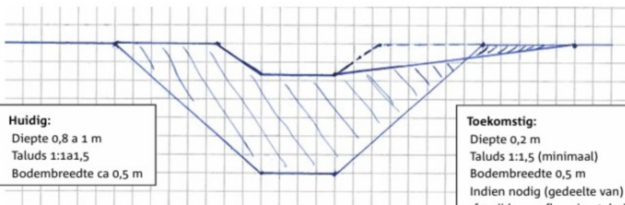
Principeprofiel verondieping
