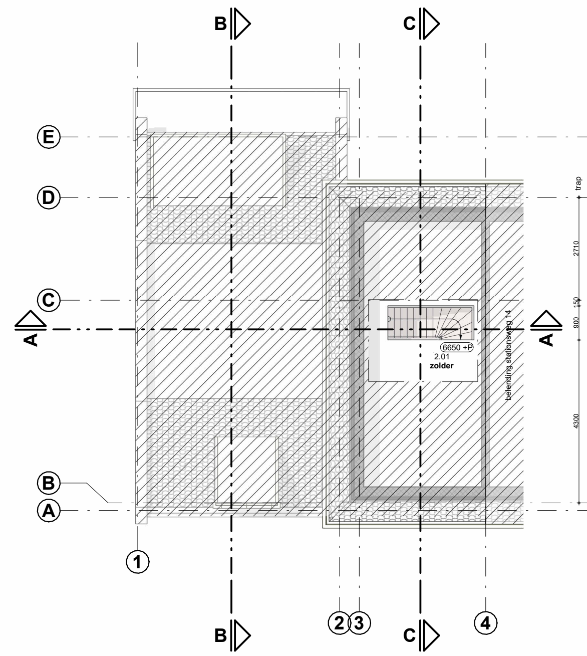
tweede verdieping
