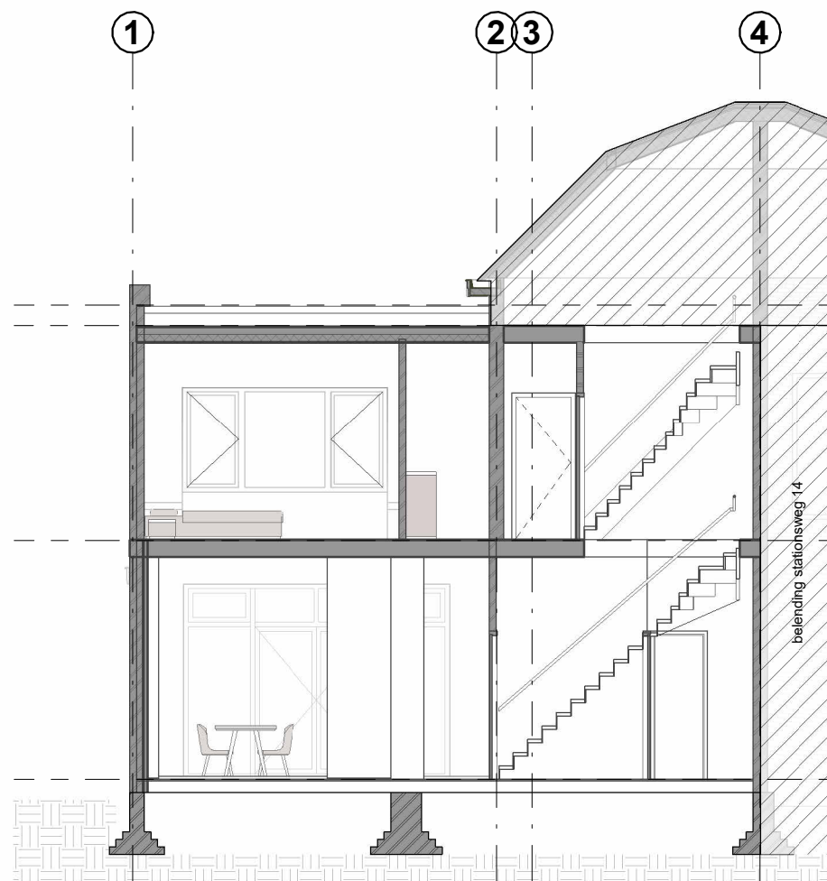
doorsnede A-A
