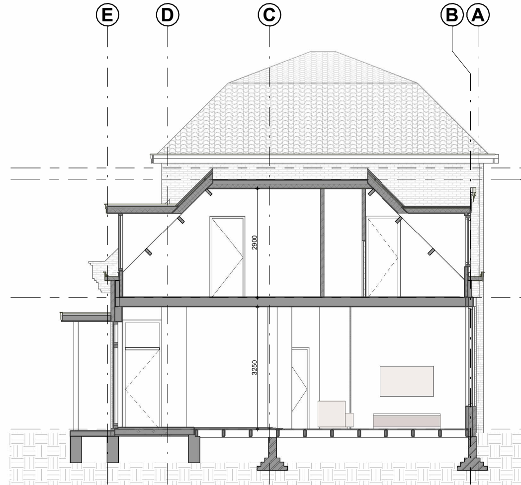
doorsnede B-B
