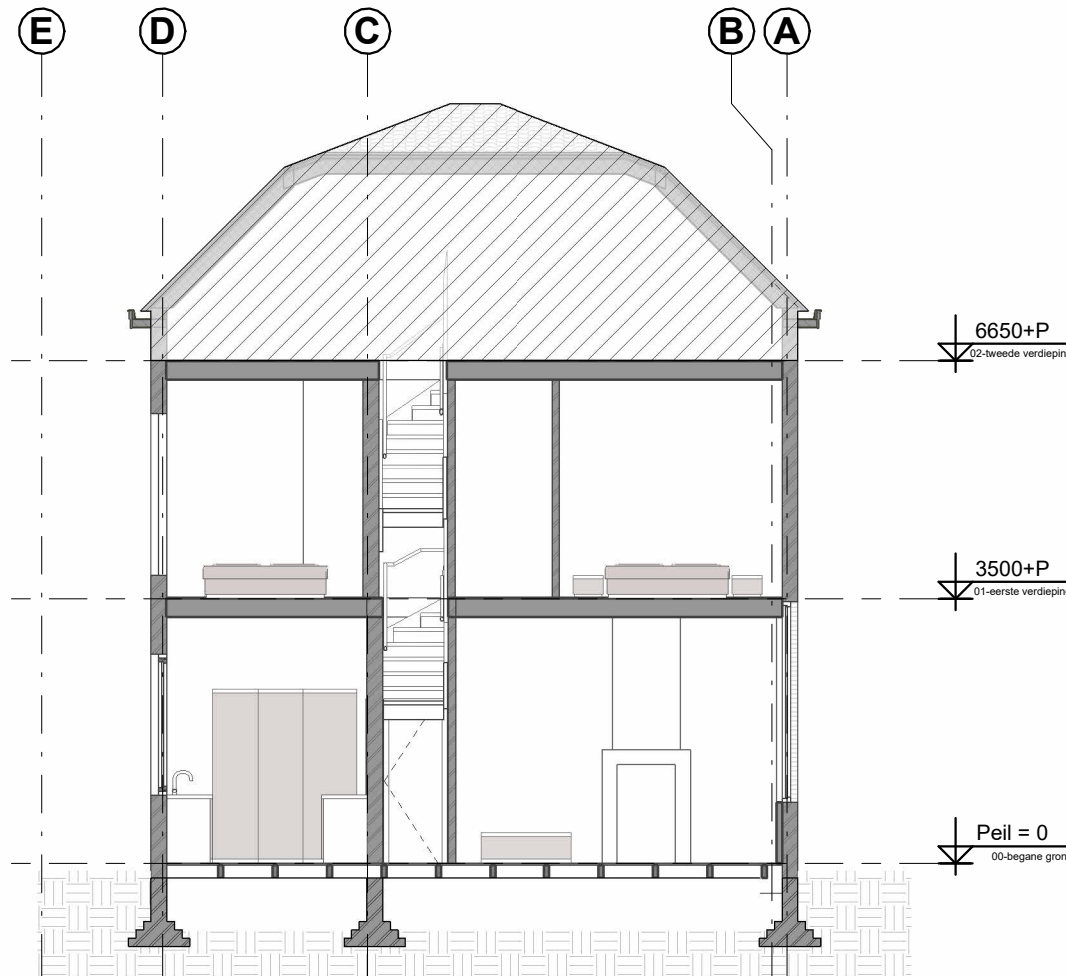
doorsnede C-C
