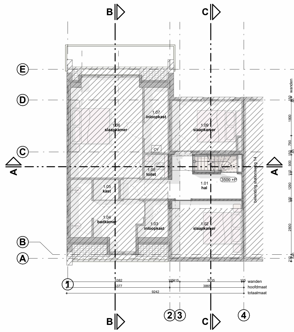
eerste verdieping
