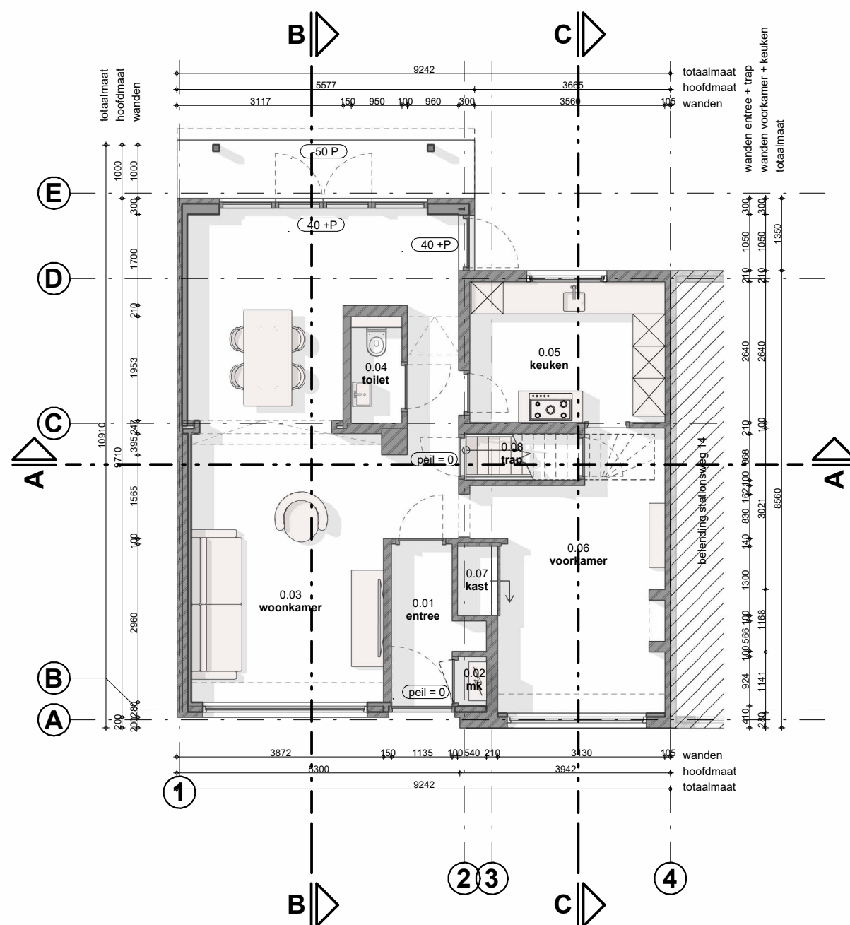
begane grond
