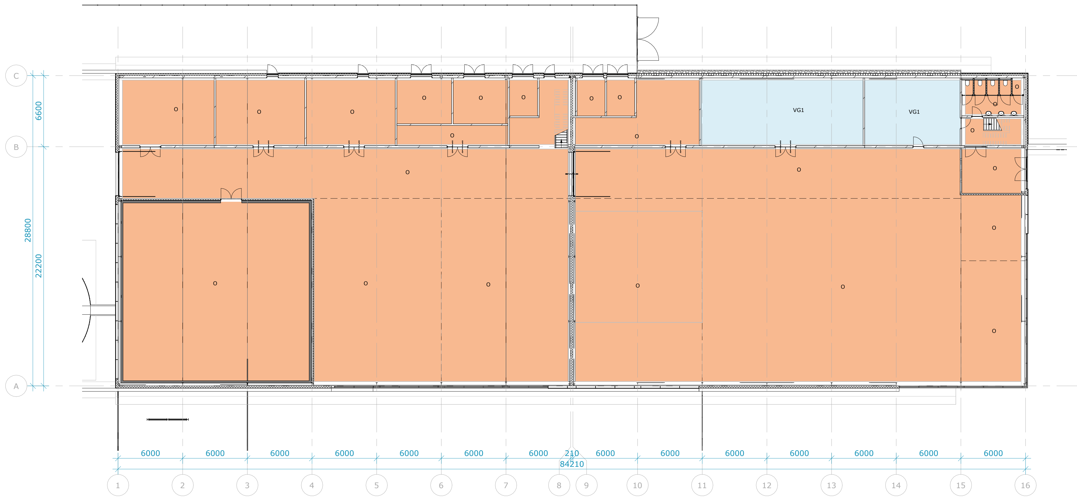
Begane grond
