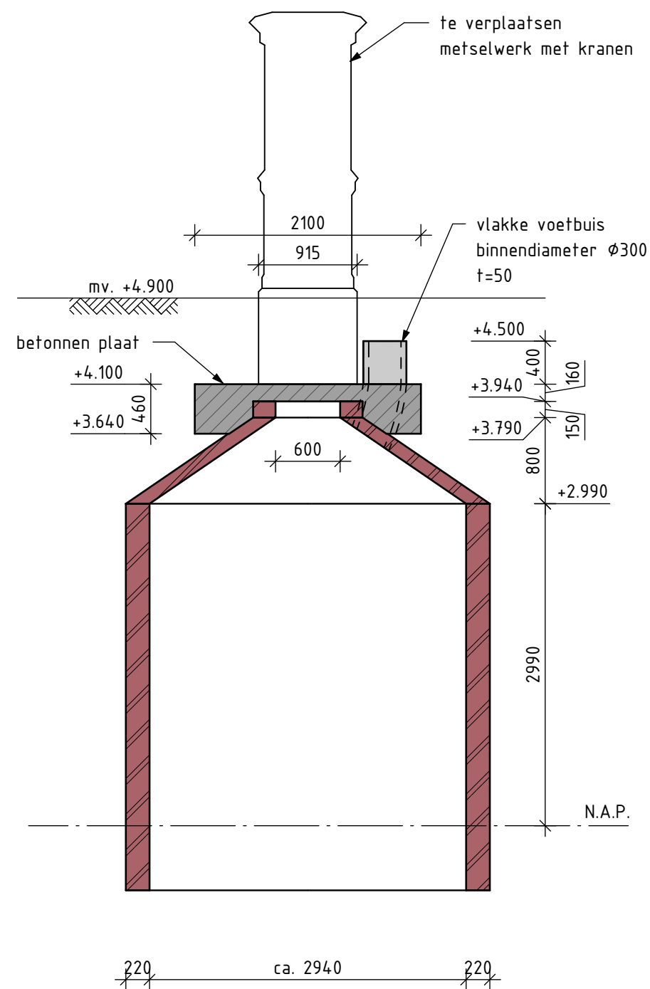
DOORSNEDE PUT schaal: 1 : 50
