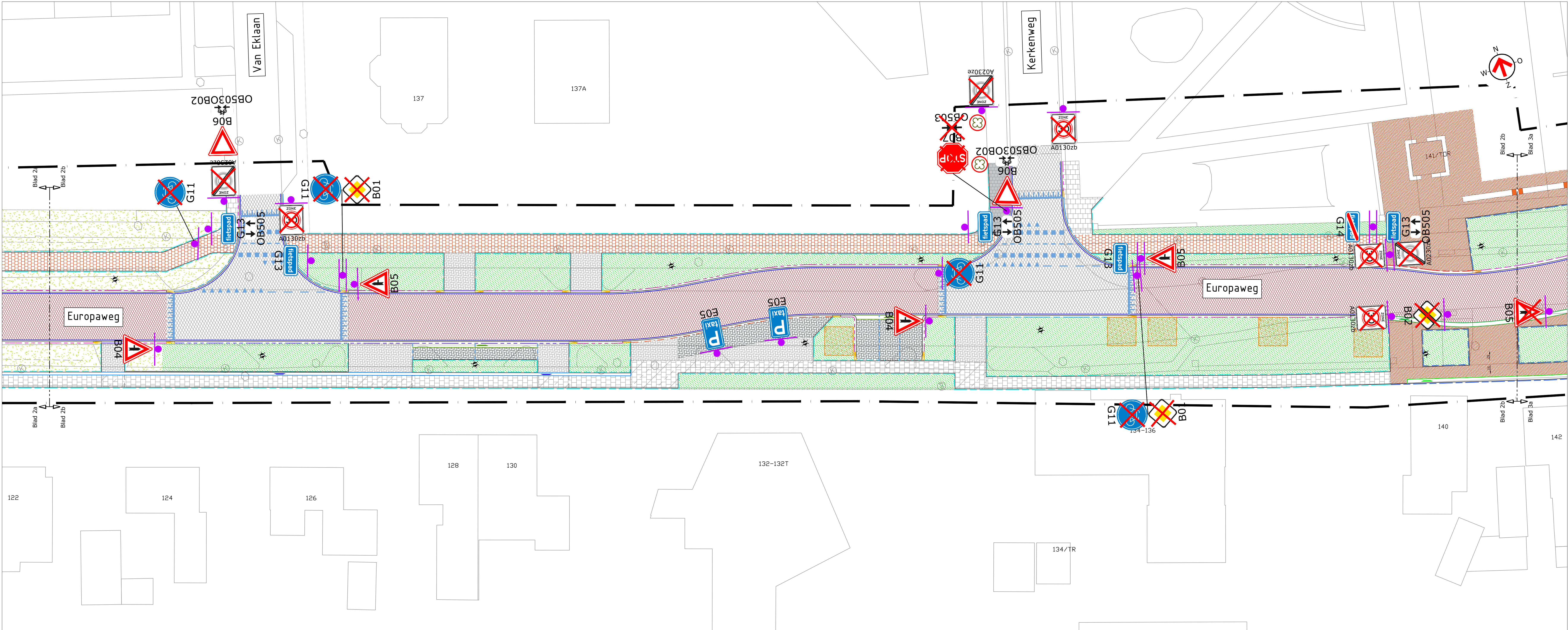
Situatie 2b SCHAAL 1:200
