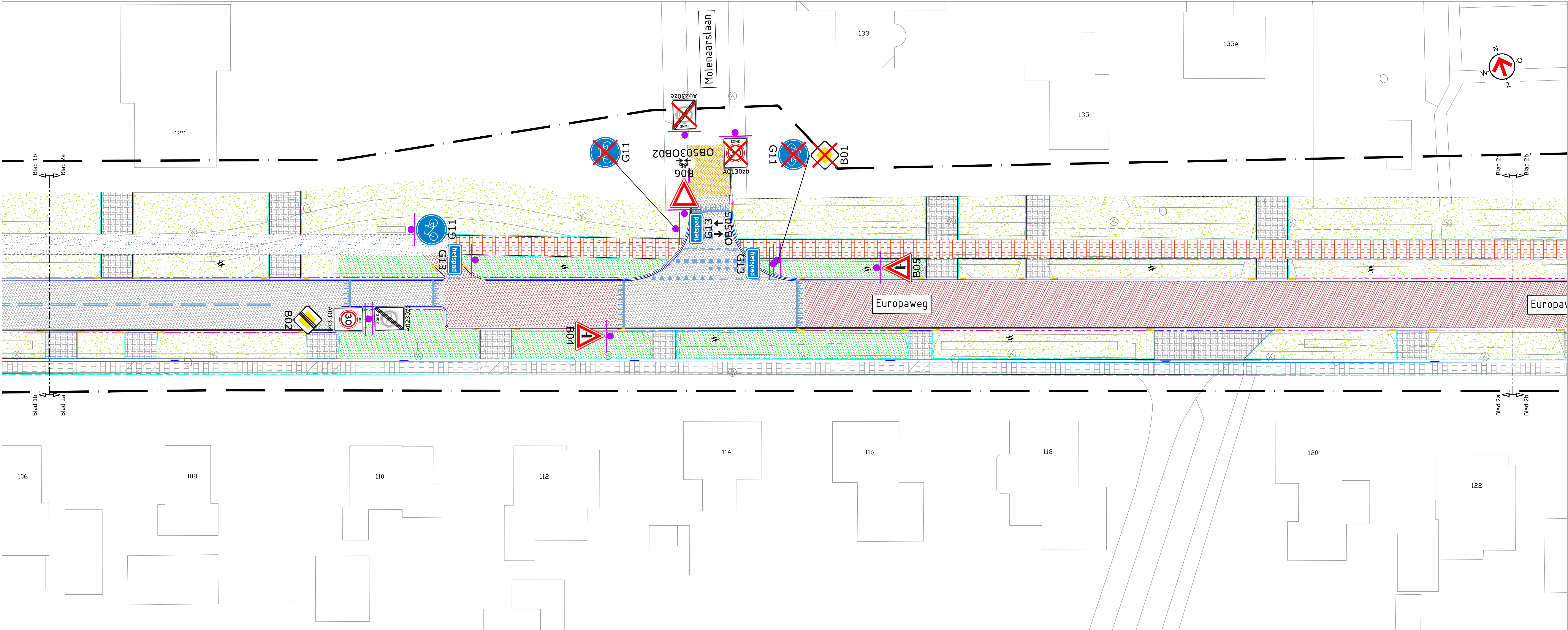
Situatie 2a SCHAAL 1:200
