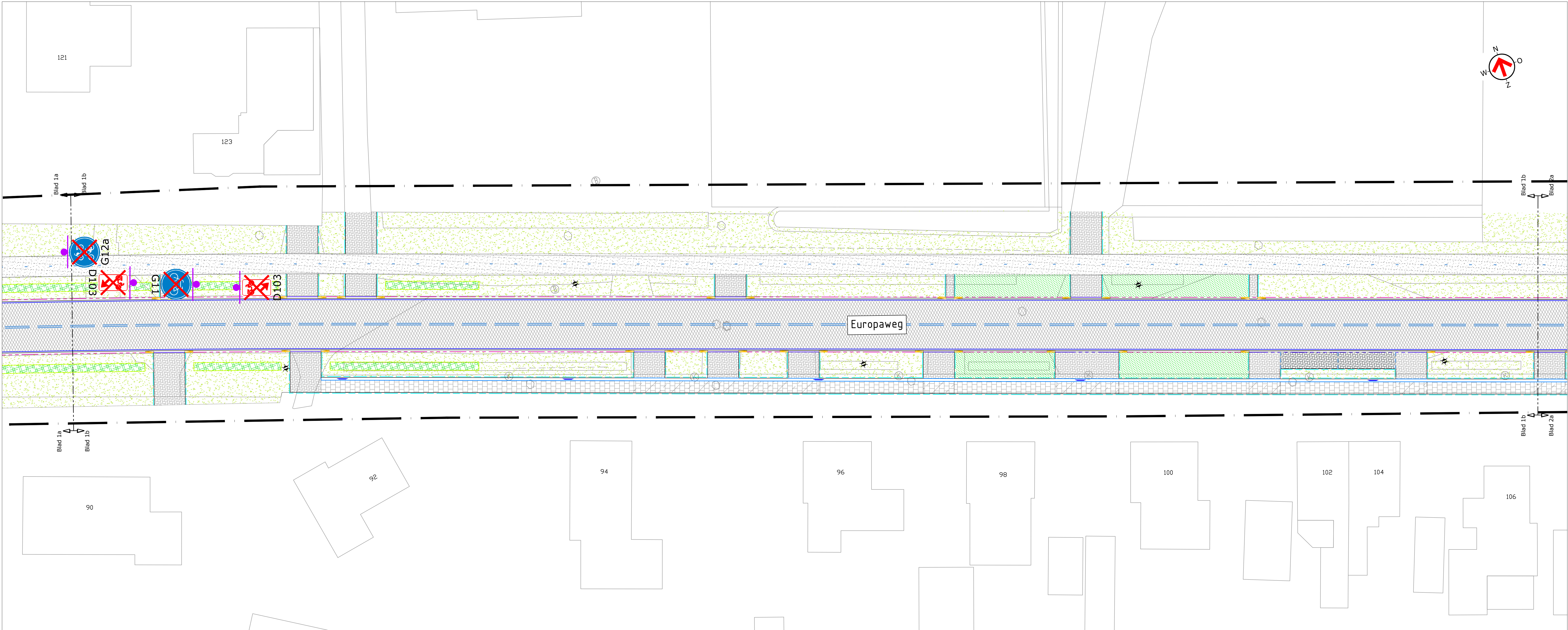
Situatie 1b SCHAAL 1:200
