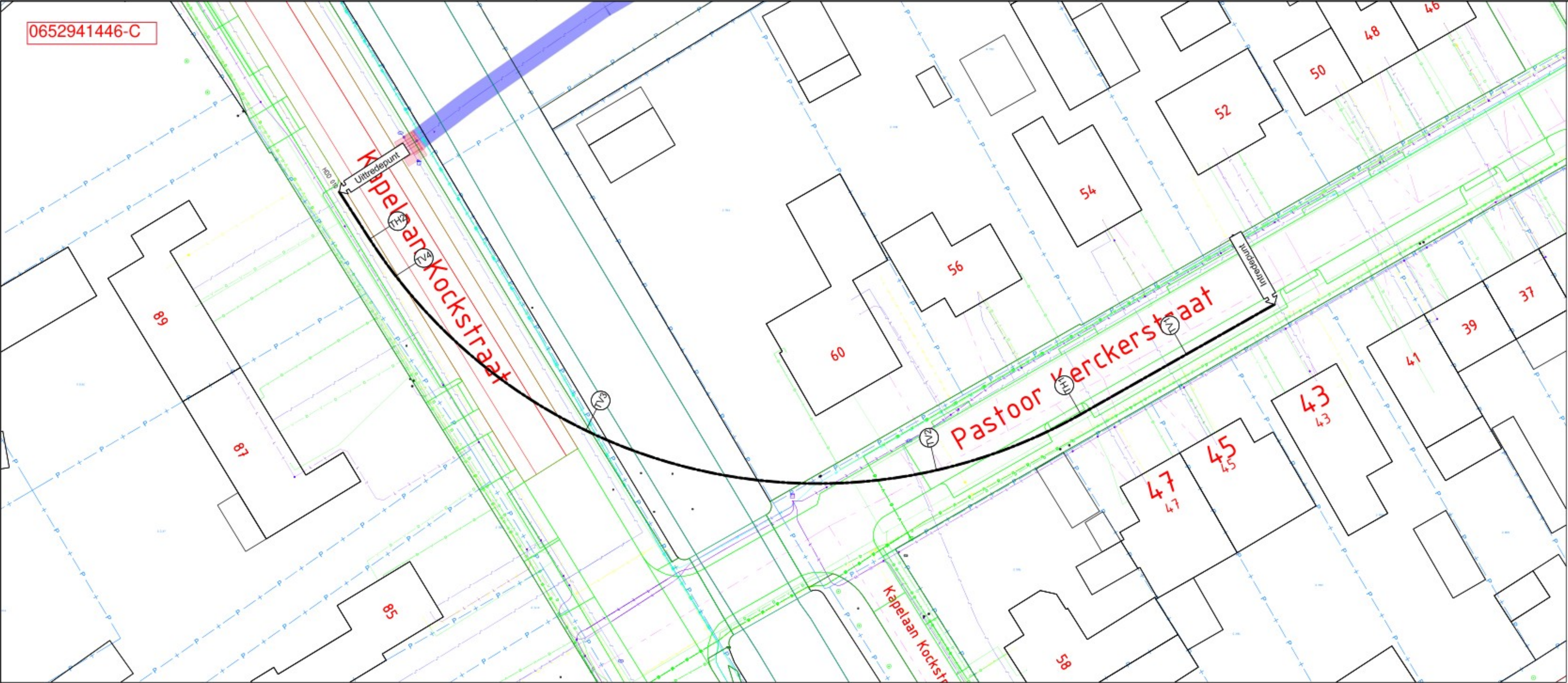
Bovenaanzicht Schaal: 1:250
