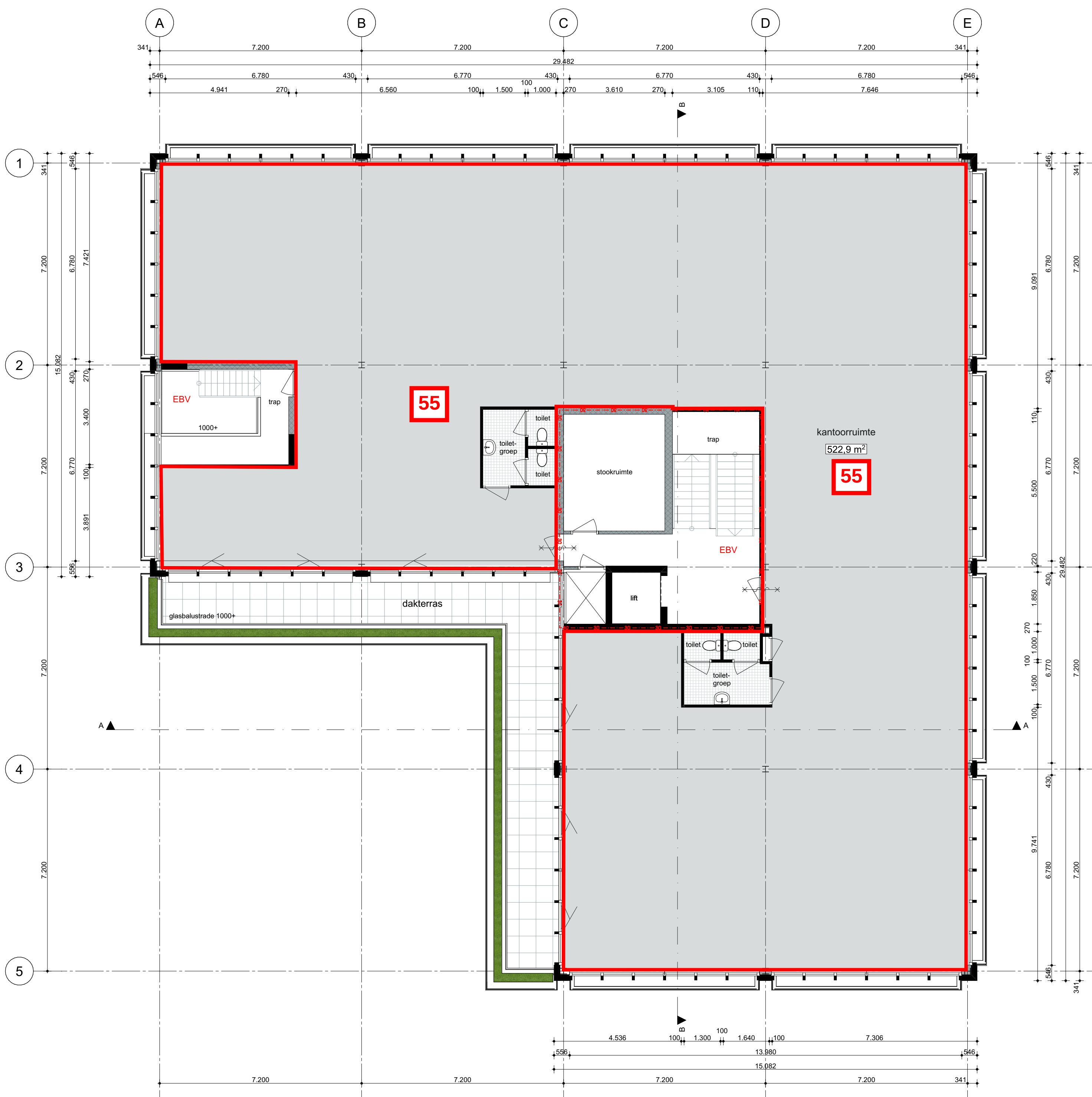
4E VERDIEPING
