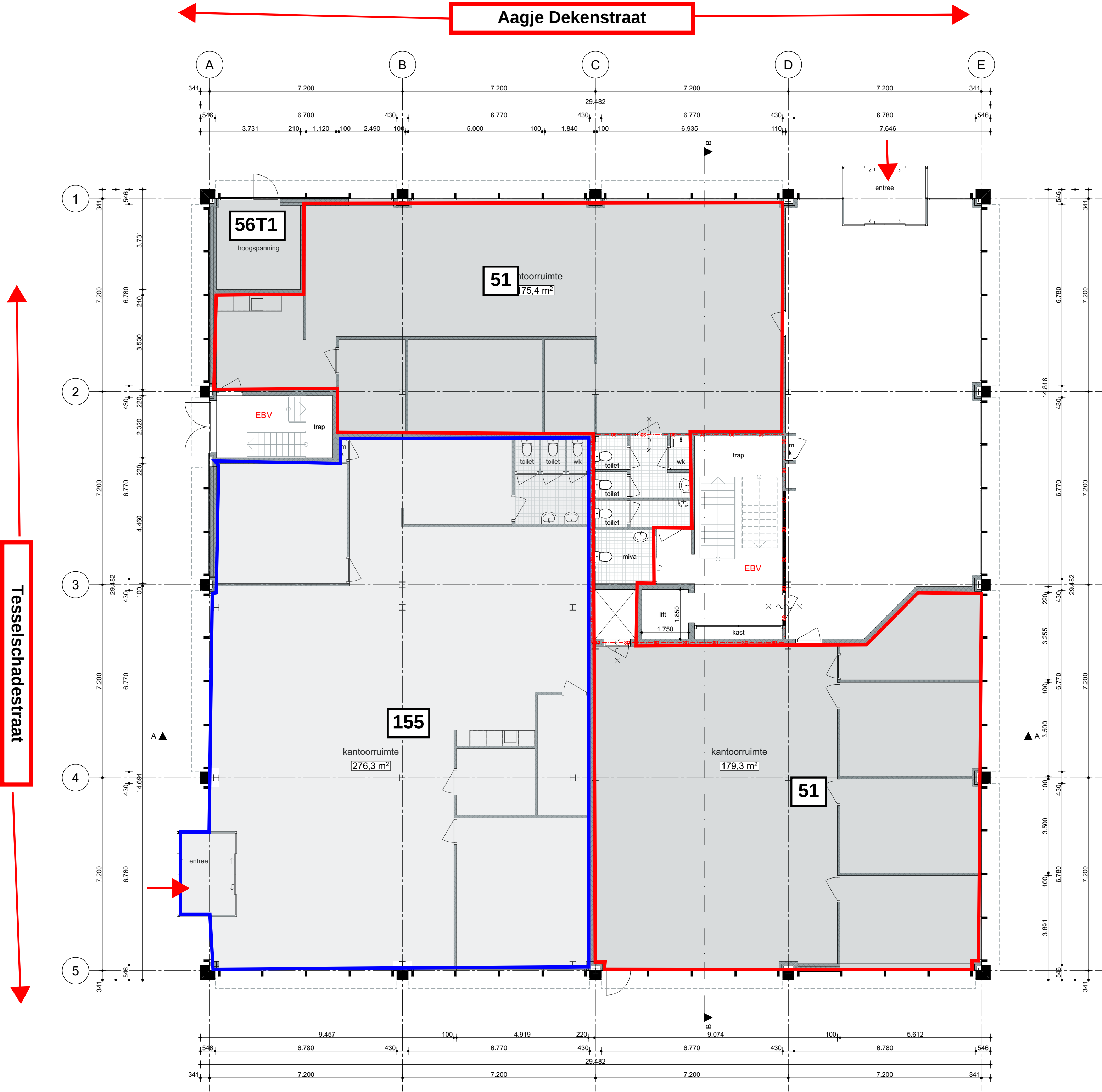
BEGANE GROND
