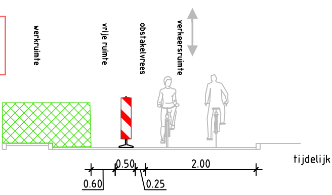
Dwarsprofiel A-A
