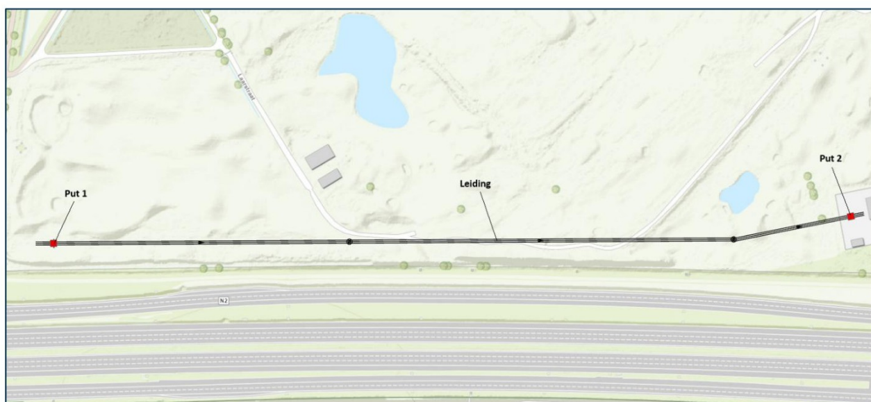
Figuur 9: Situering rioolvoorzieningen.
