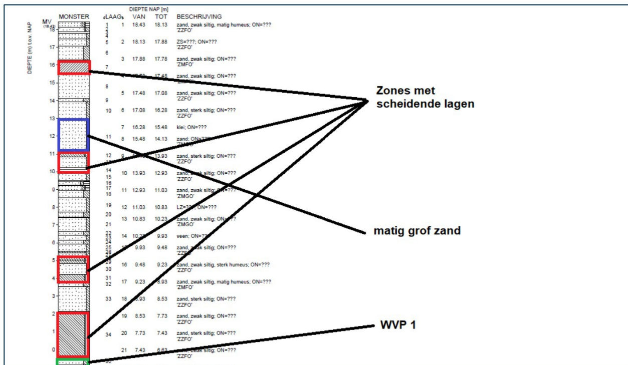
Figuur 4: Representatieve bodempopbouw tracé.
