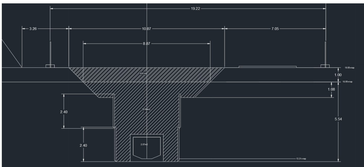
Figuur 10: Principedetail sleuven.
