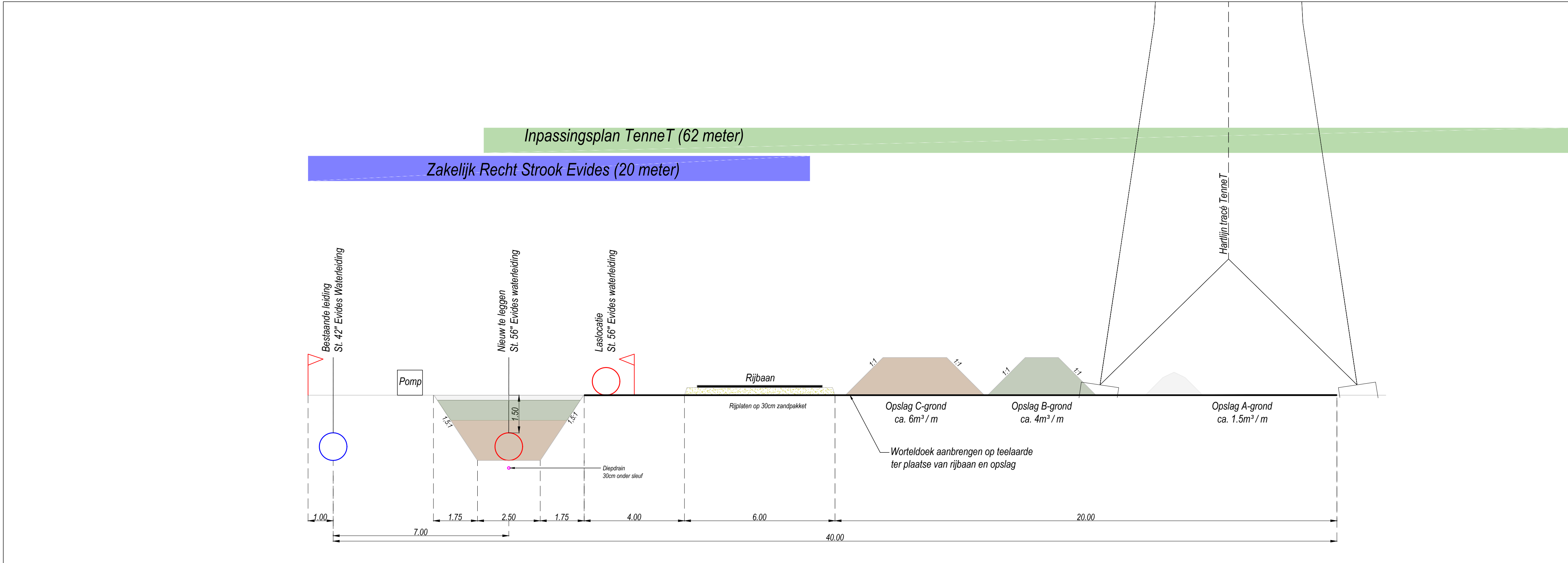
Doorsnede B-B: Principe detail Werkstrook Schaal 1:100
