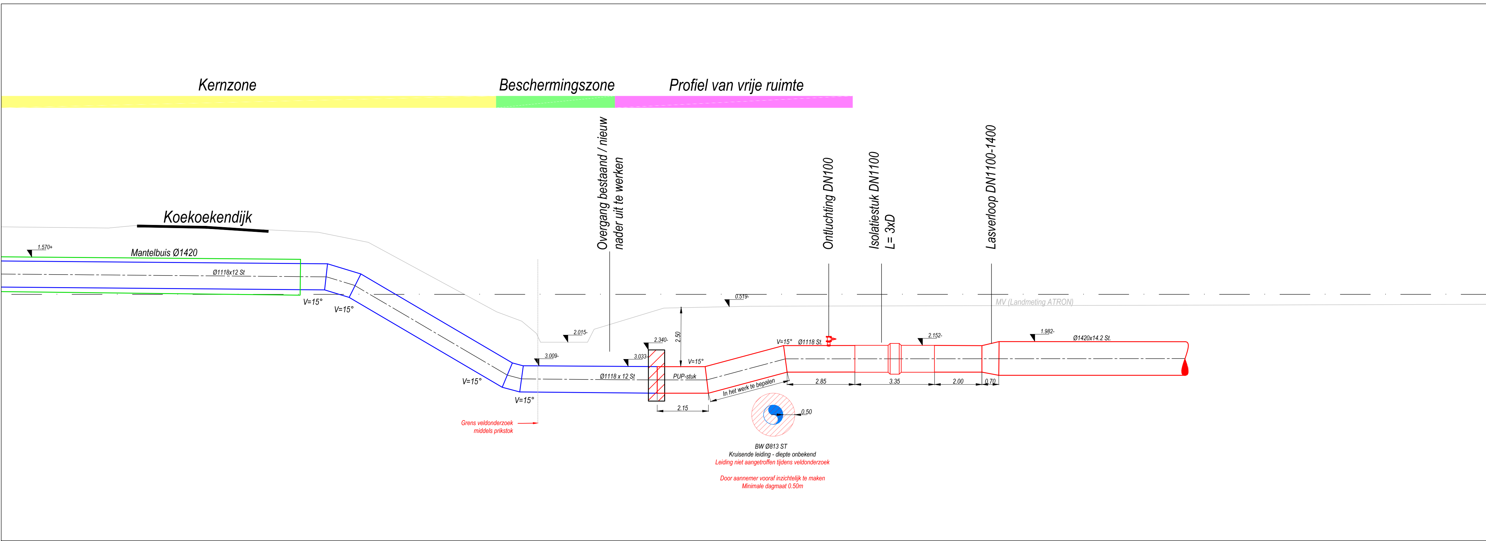
Doorsnede 1-1 Aansluiting Koekoekendijk Schaal 1:100
