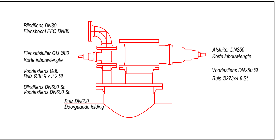
Detail mangat - opbouw type A Schaal 1:20
