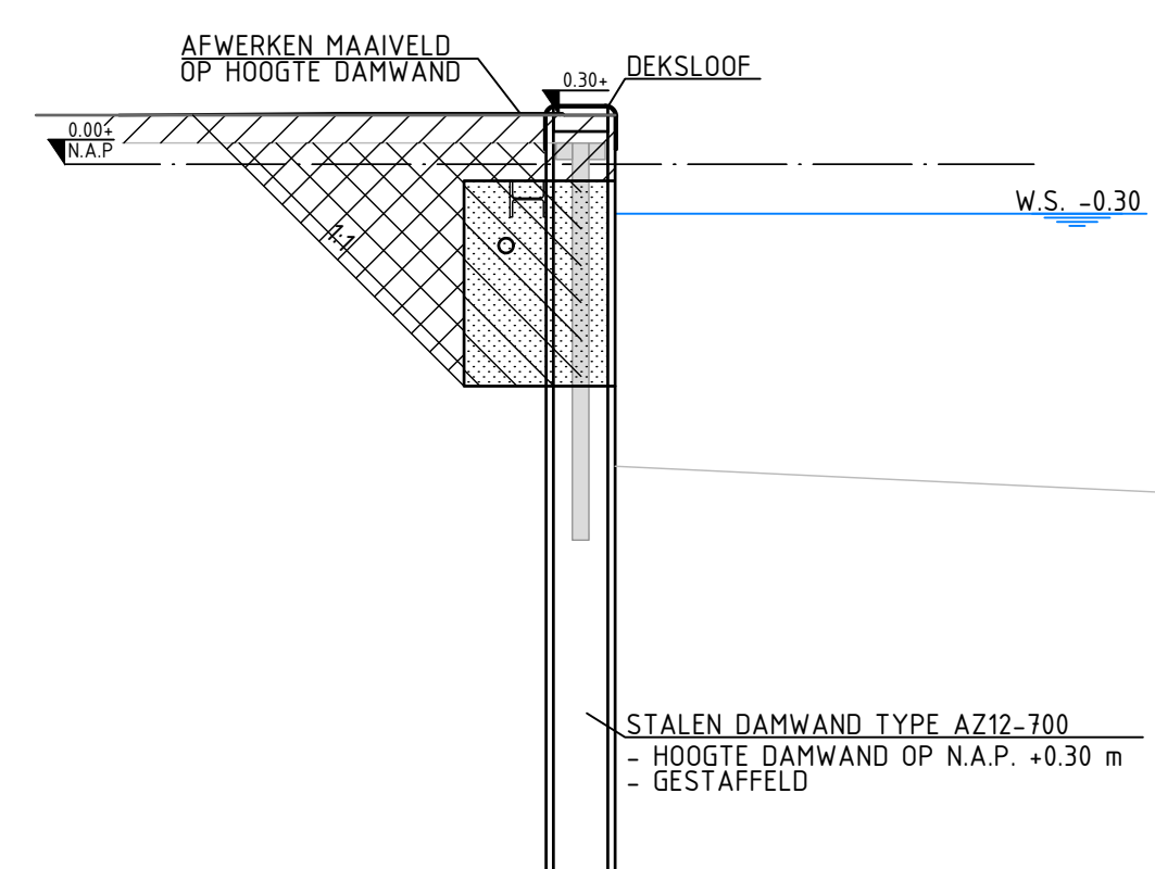
DETAIL 2 STALEN DAMWAND HAKKELAARSBRUG 2 - 5 SCHAAL 1 : 50
