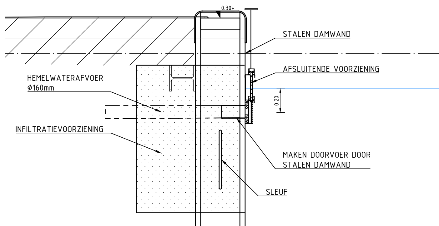
DETAIL 4 AFSLUITER HEMELWATER SCHAAL 1 : 20
