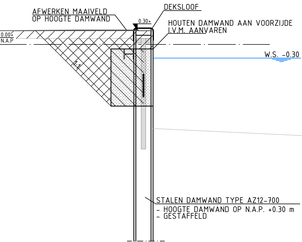
DETAIL 1 STALEN DAMWAND HAKKELAARSBURG 1 SCHAAL 1 : 50
