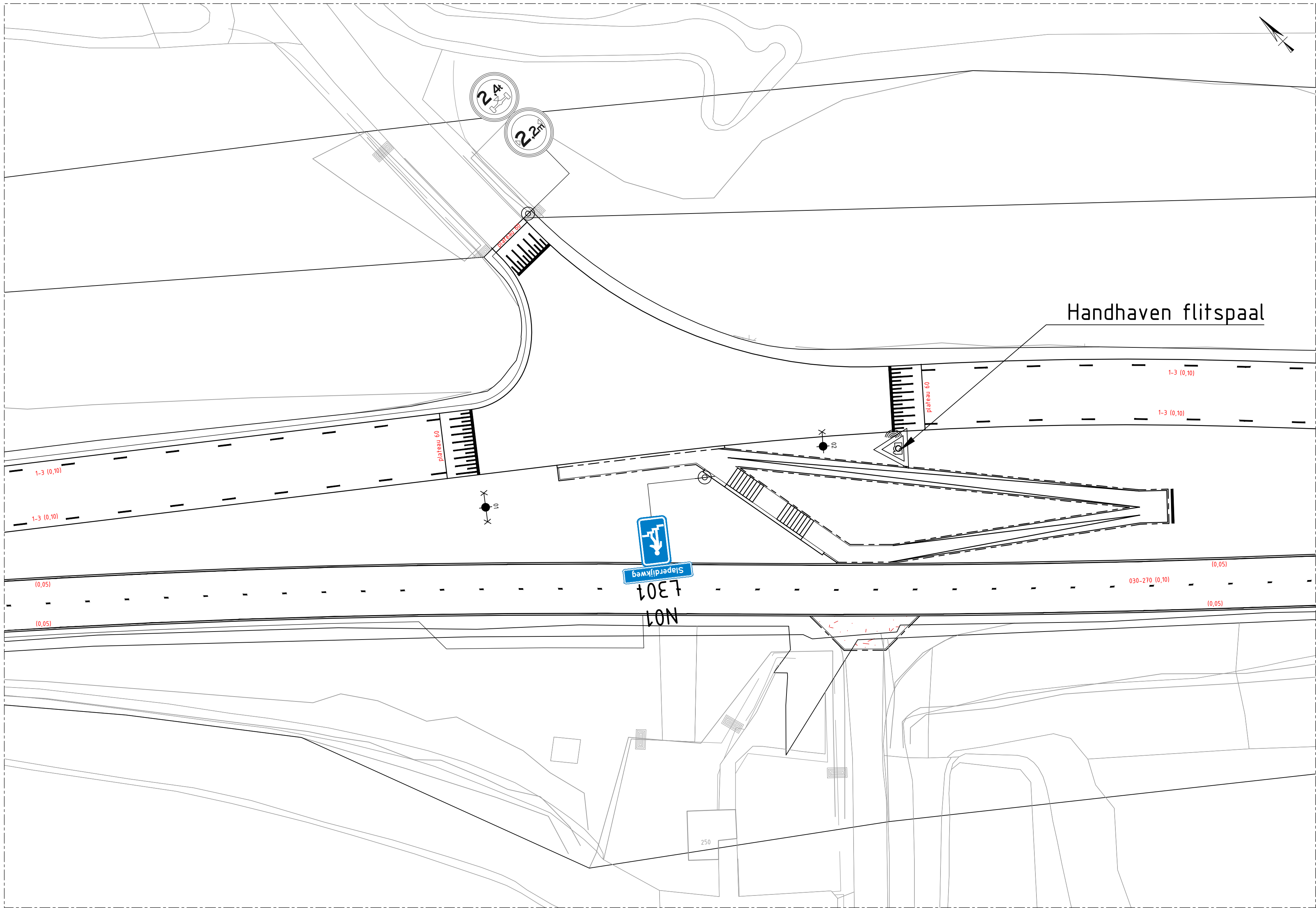
SITUATIE: KRUISING WESTLAAN Schaal 1:200
