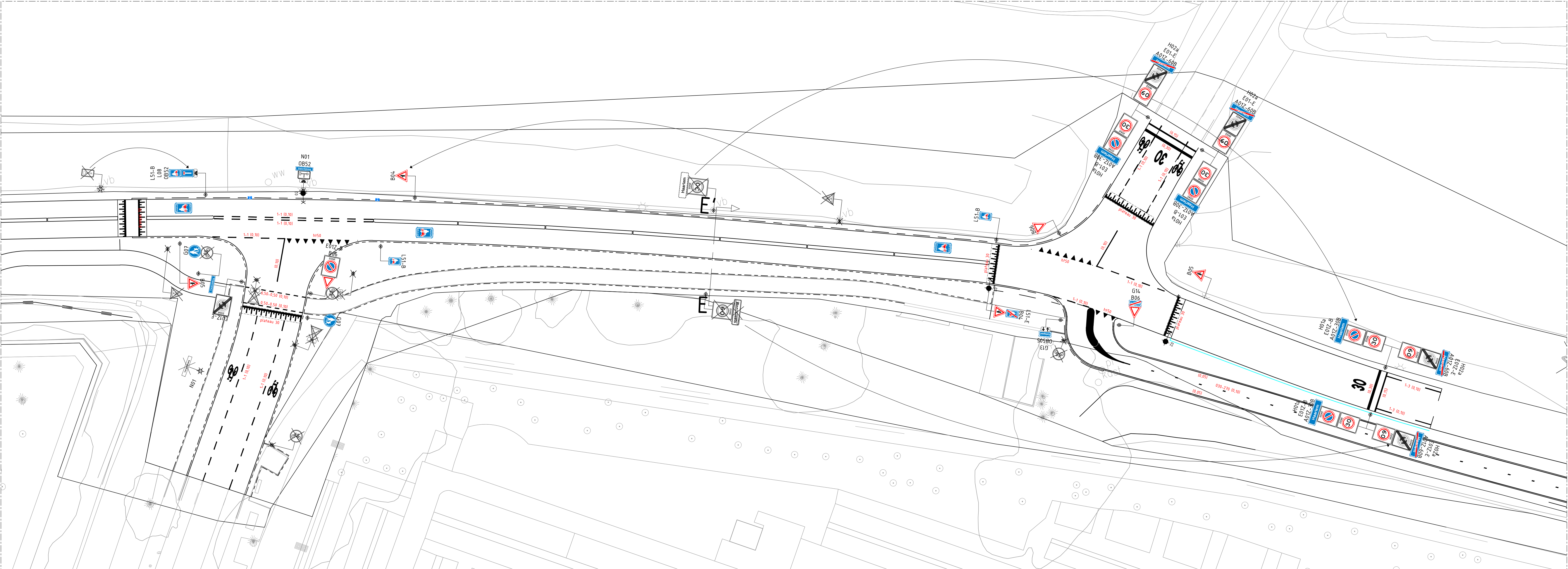
SITUATIE: KRUISING VERGIERDEWEG - OOSTLAAN Schaal 1:200
