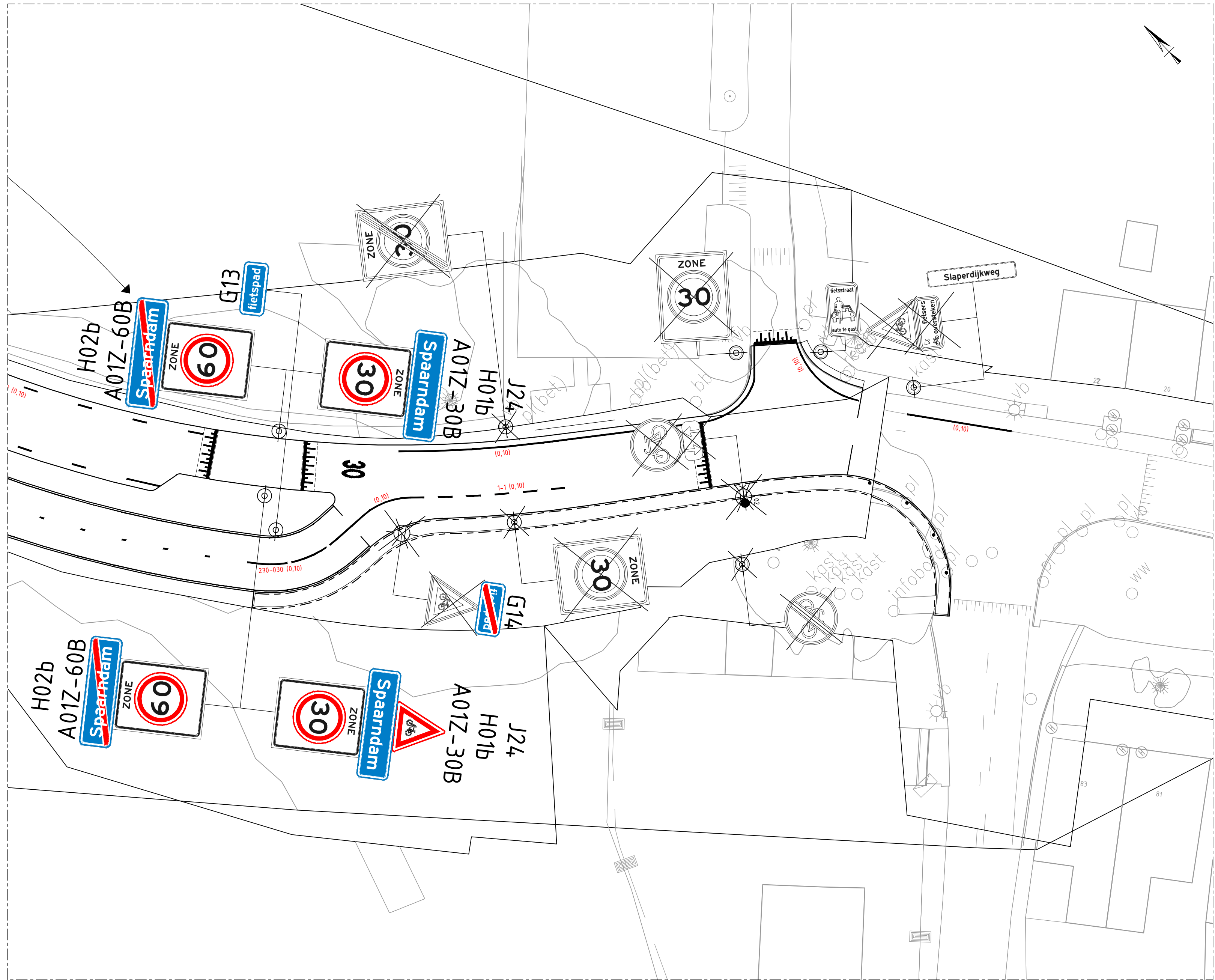
SITUATIE: KRUISING REDOUTE - NIEUWE RIJWEG Schaal 1:200
