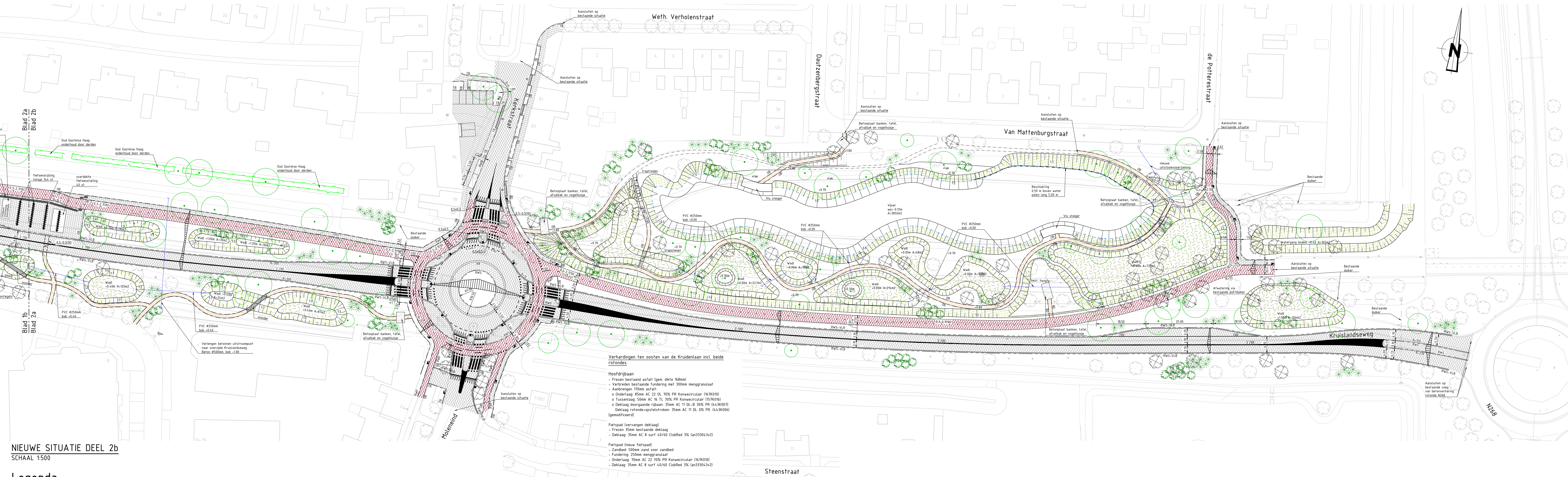
NIEUWE SITUATIE DEEL 2b SCHAAL 1:500
