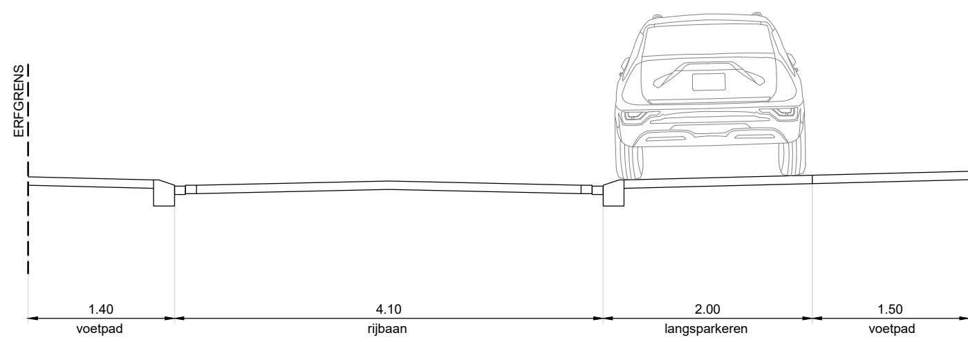
Principe profil bestaande situatie Situering: ter plaatse van parkeren naast rijbaan Schaal 1:50
