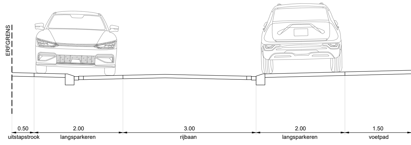
Principe profil nieuwe situatie Situering: ter plaatse van parkeren op trottoir/rijbaan Schaal 1:50
