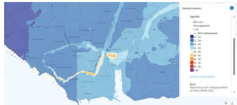
Afbeelding 11: Jaargemiddelde concentratie stikstofdioxiden (NO 2 ) in 2022.
