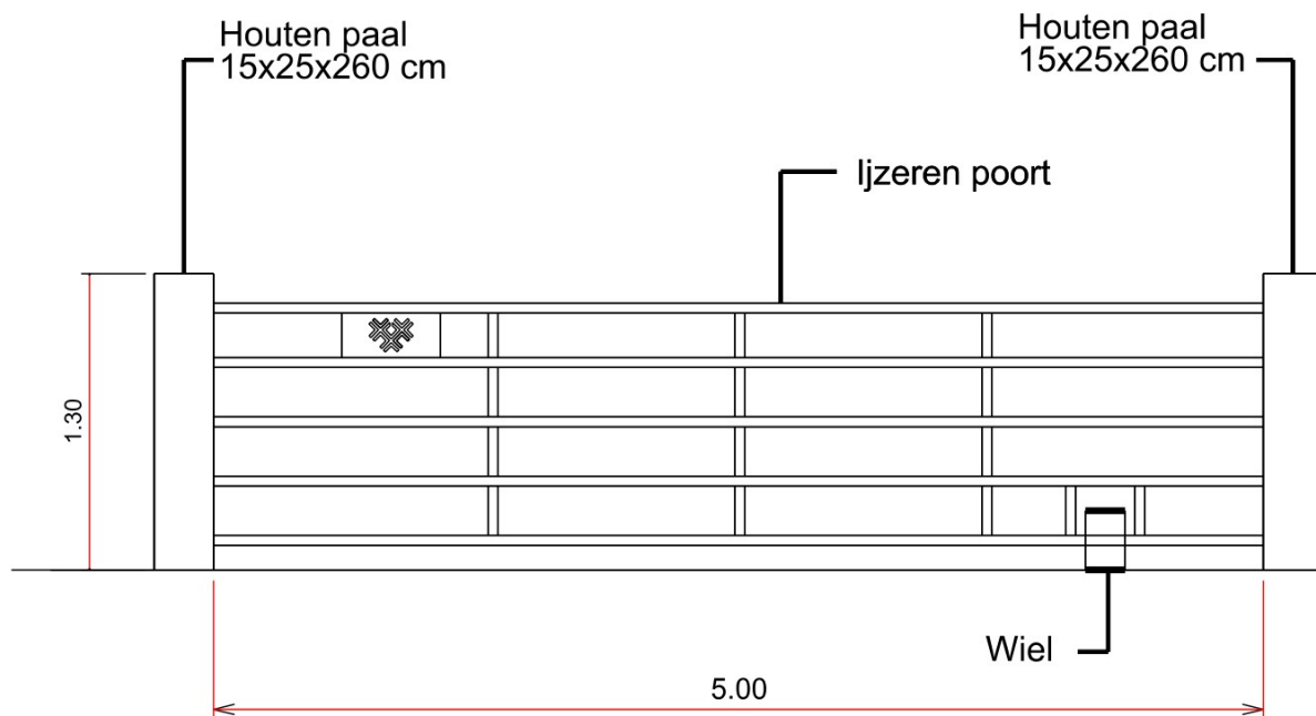
DETAIL ONDERHOUDSPOORT
