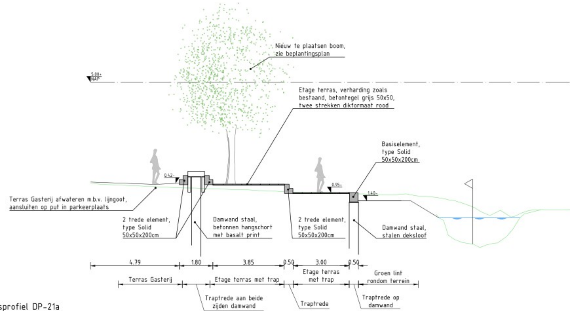
Dwarsprofiel DP-21a
