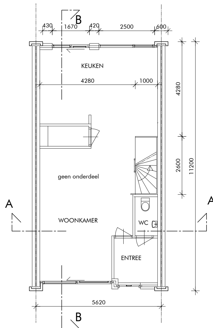
BEGANE GROND
