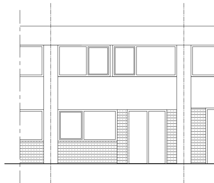
ACHTERGEVEL
