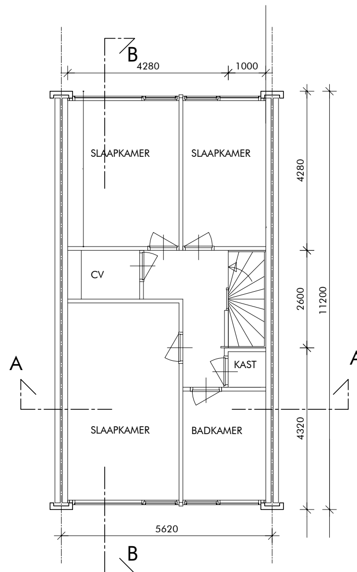
1e VERDIEPING
