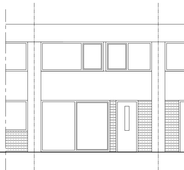
VOORGEVEL
