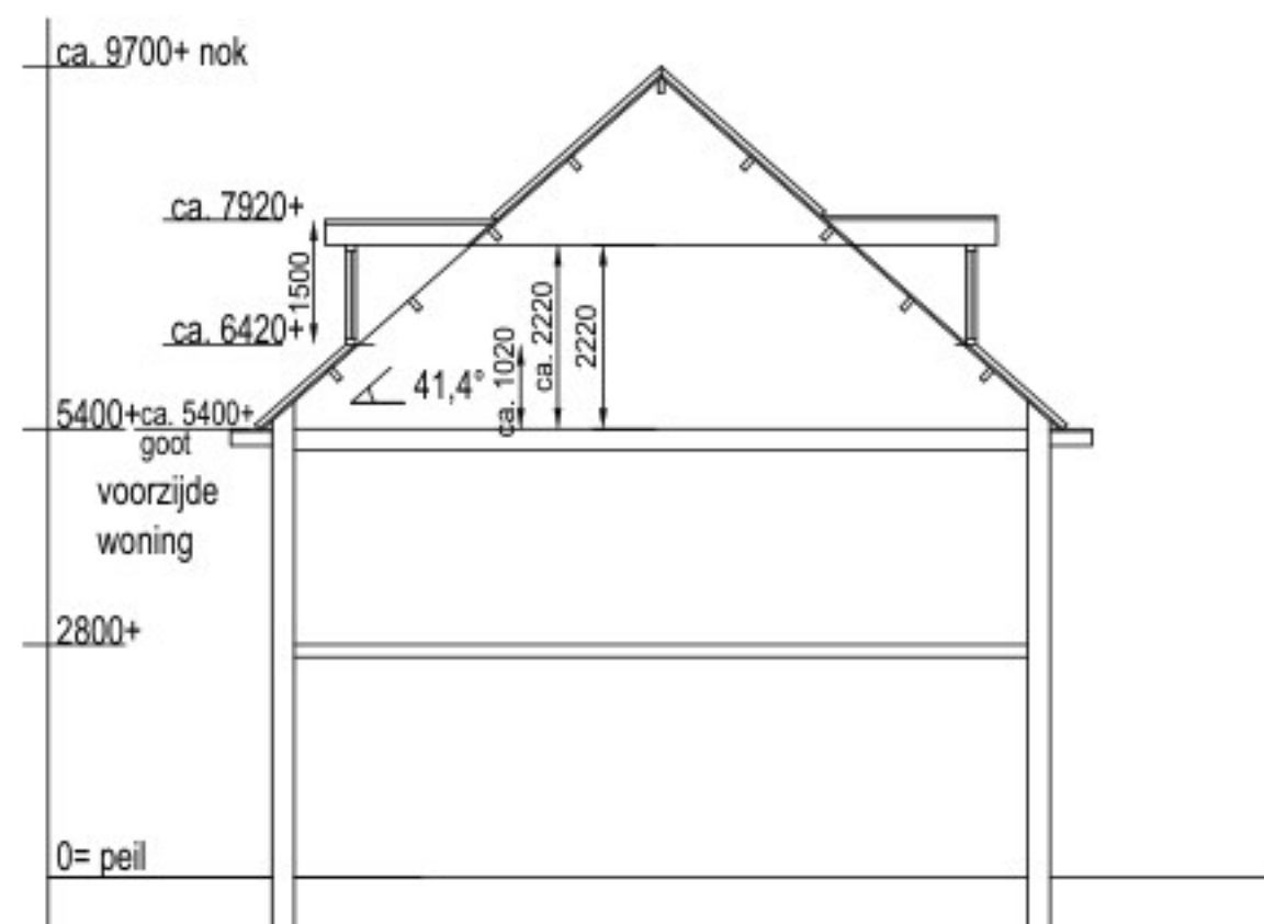
doorsnede nieuw
