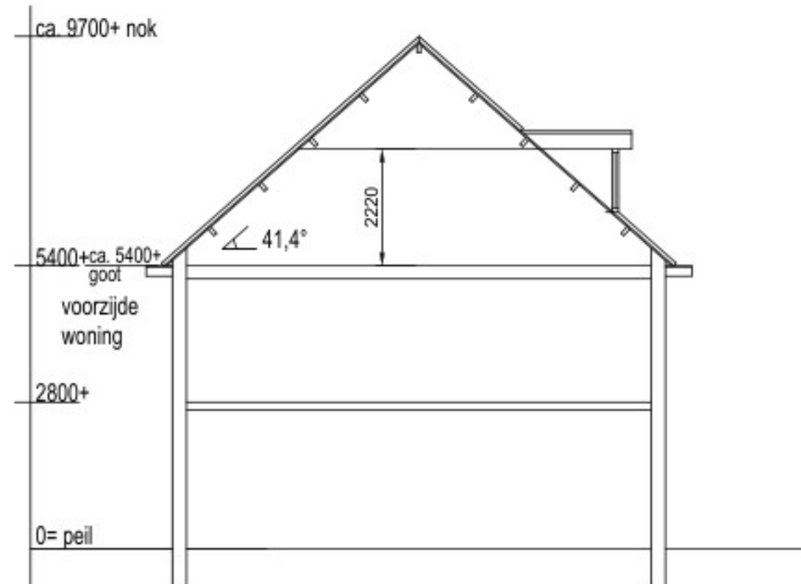
doorsnede bestaand
