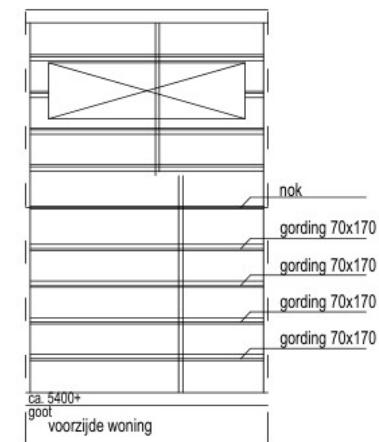
kapplan bestaand
