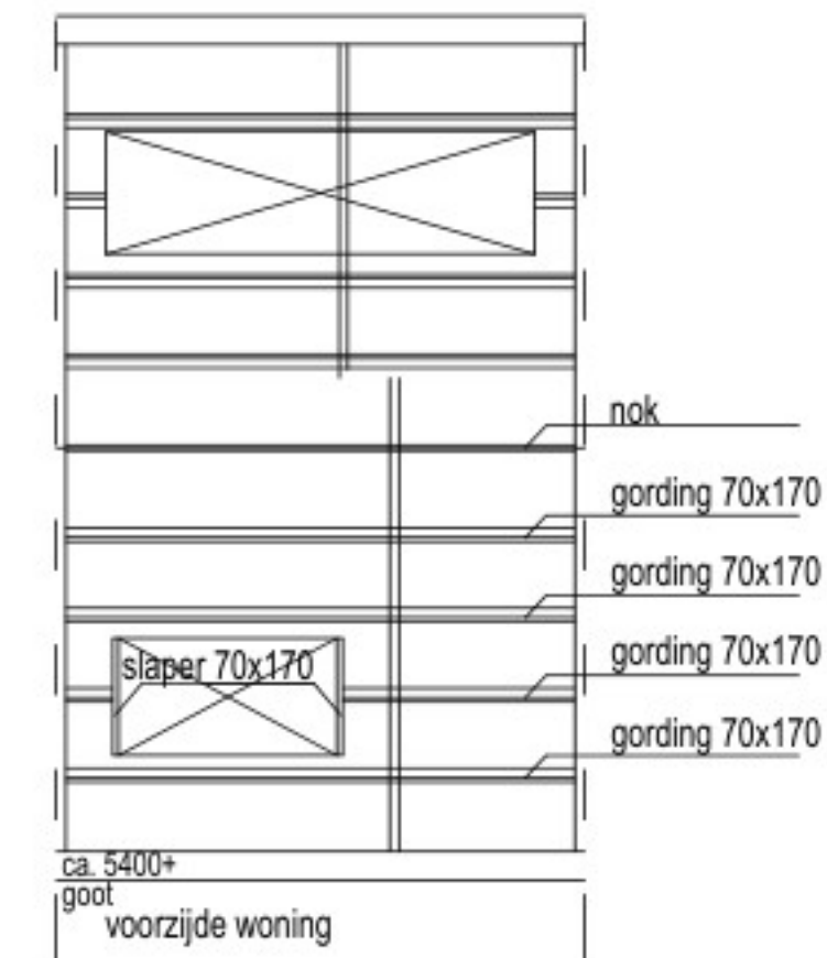
kapplan nieuw
