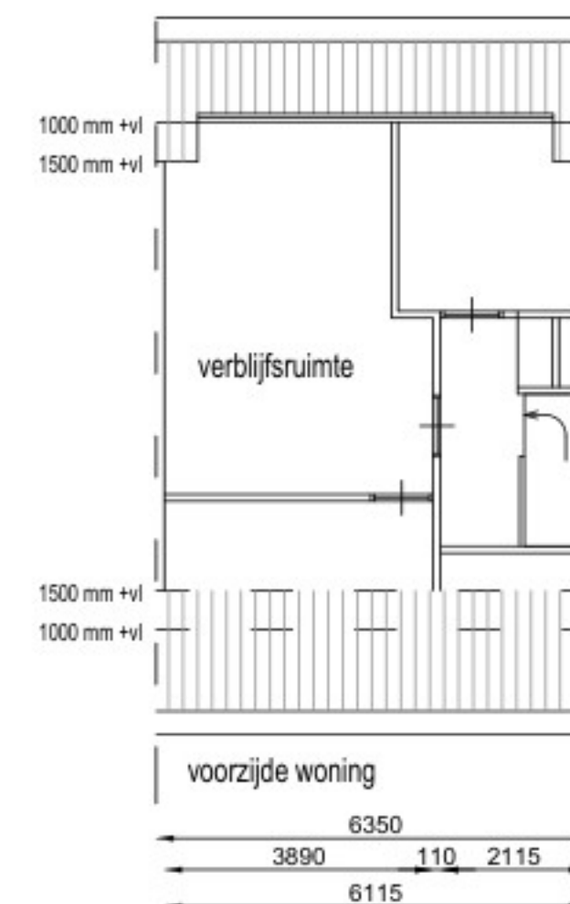
indeling bestaand
