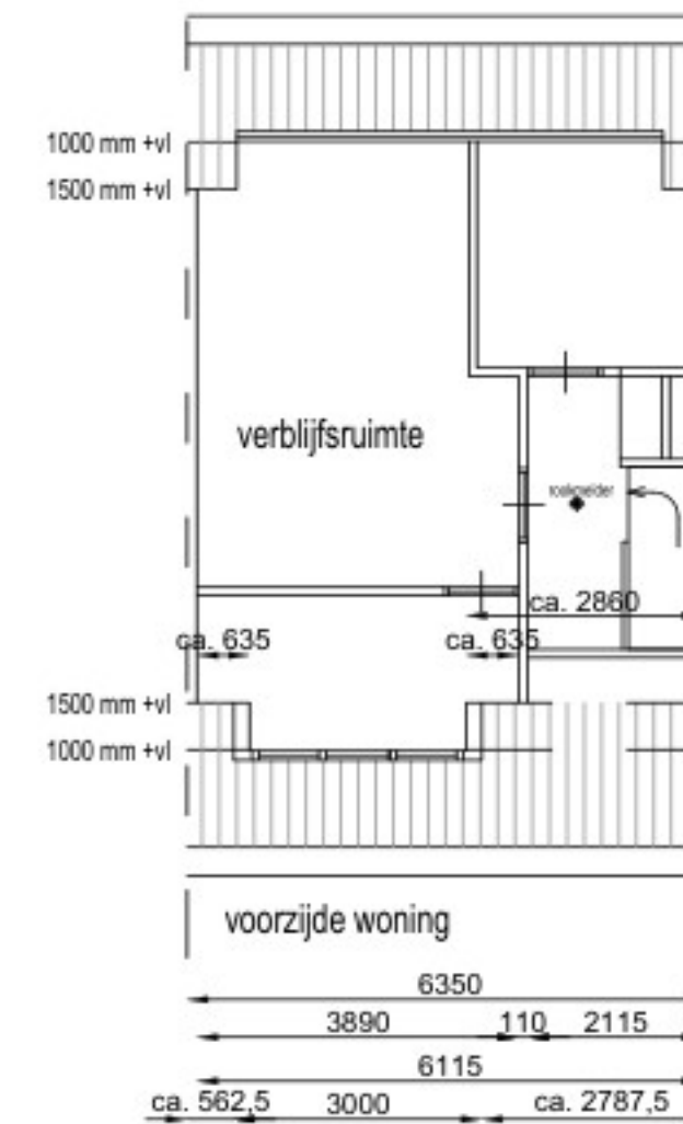
indeling nieuw
