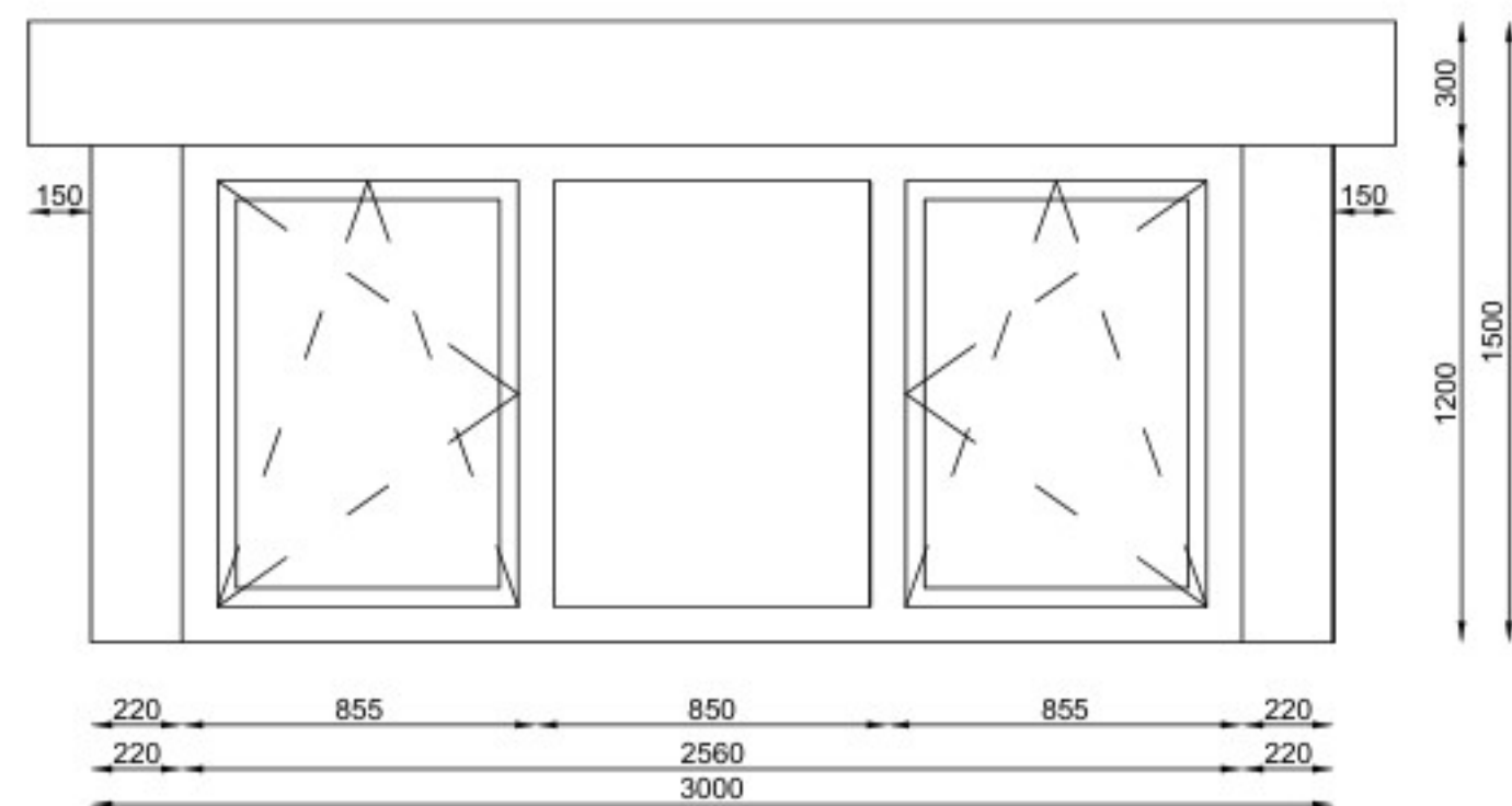
aanzicht dakkapel voorgevel schaal 1:20 type: Klassiek
