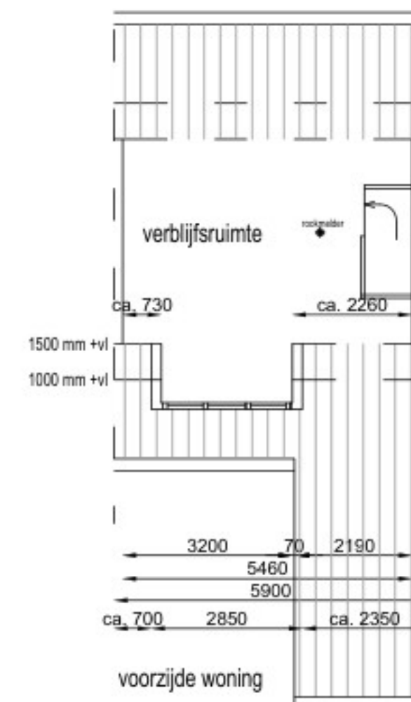
indeling nieuw
