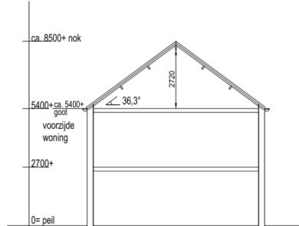
doorsnede bestaand
