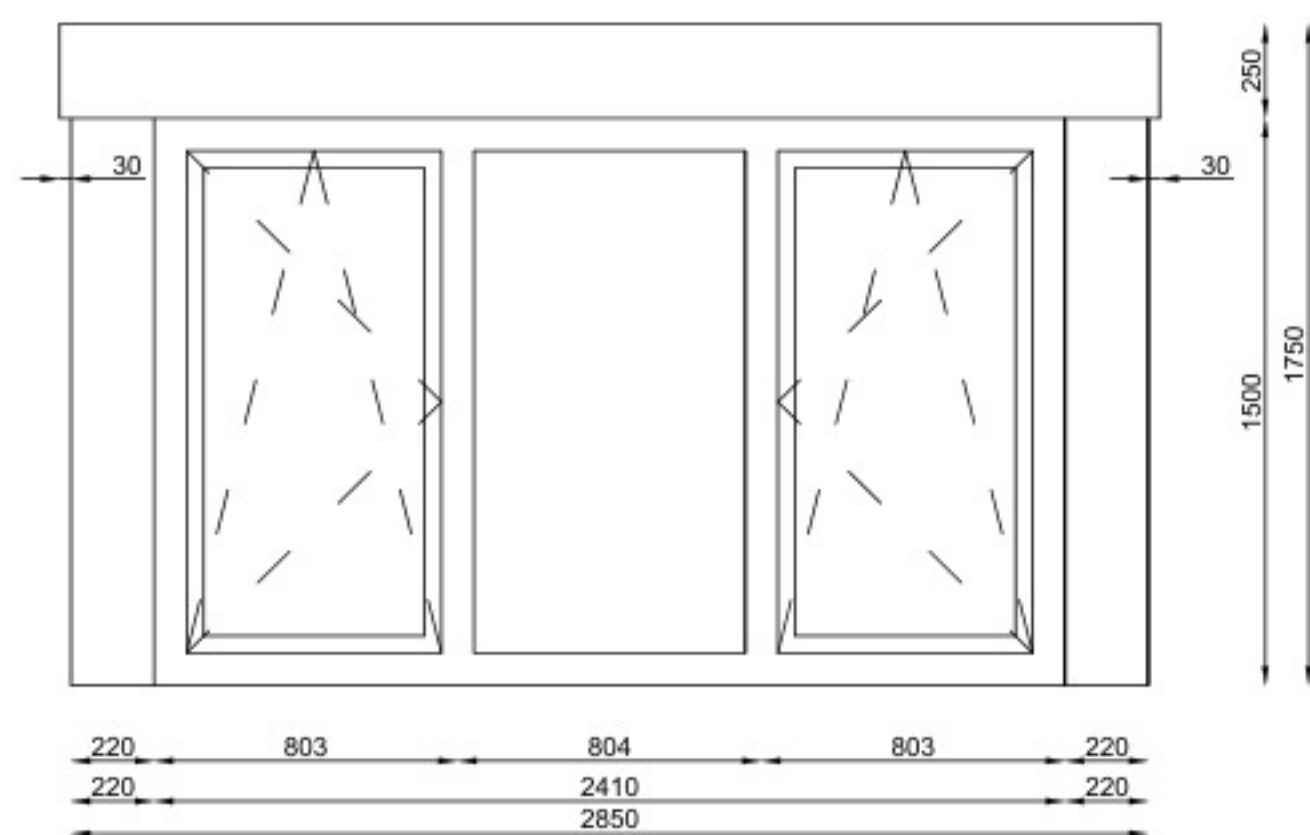
aanzicht dakkapel voorgevel schaal 1:20 type: Klassiek
