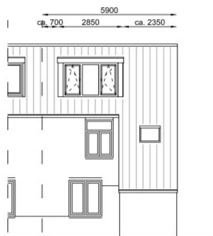
voorgevel nieuw
