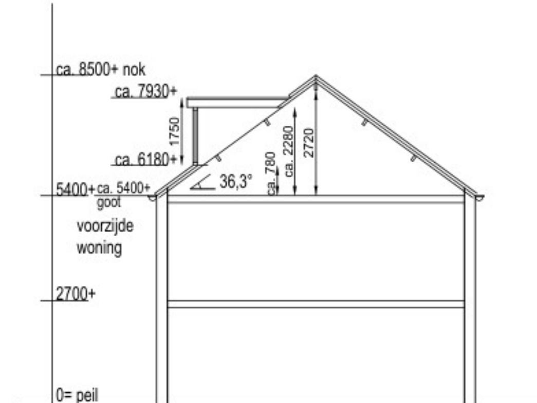
doorsnede nieuw
