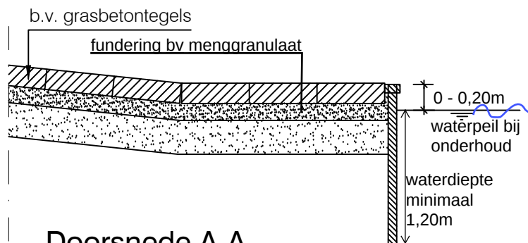
Doorsnede A-A Inlaatplaats - detail
