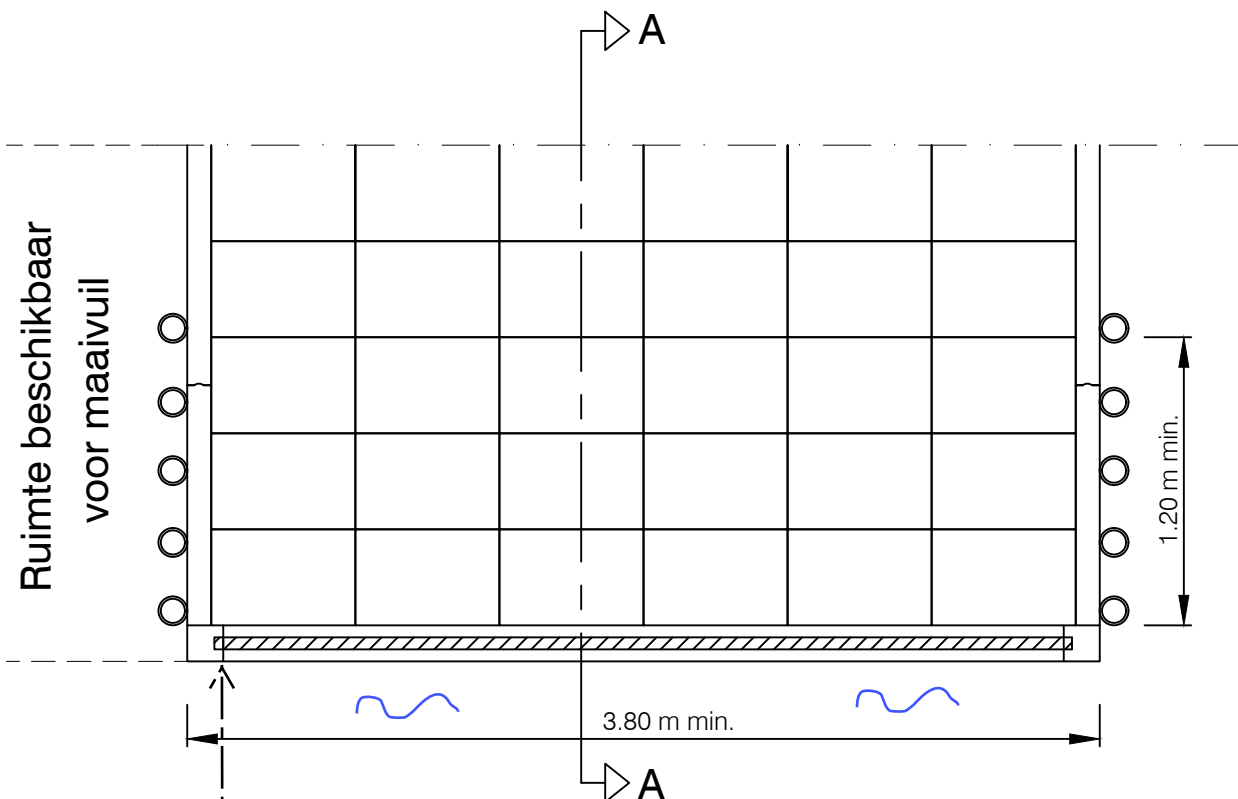
Bovenaanzicht inlaatplaats
