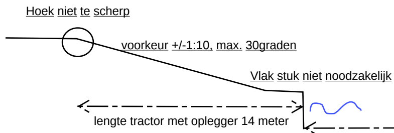
Dwarsdoorsnede inlaatplaats
