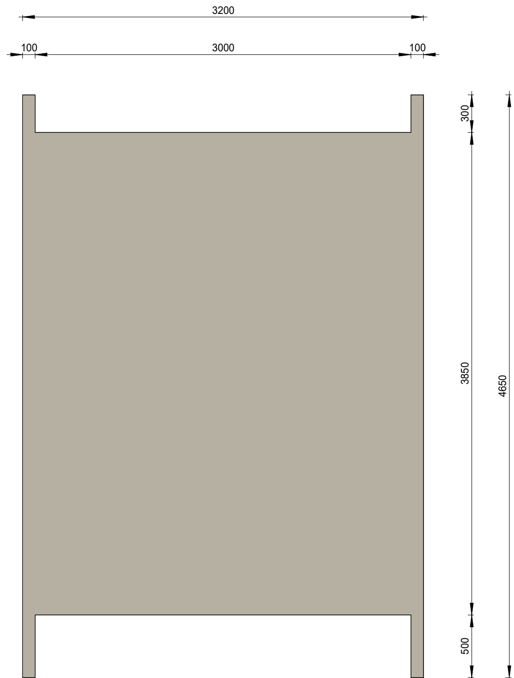
VLOERPLAAT BOVENAANZICHT
