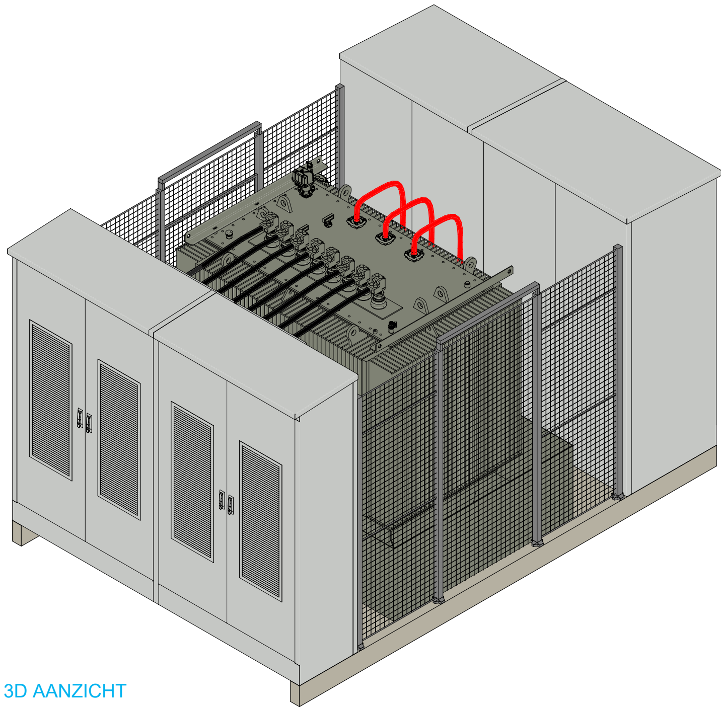
3D AANZICHT
