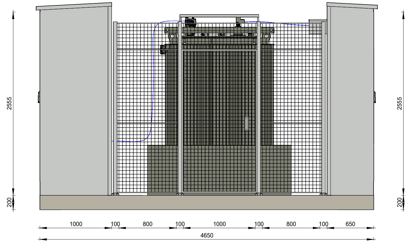
LINKER ZIJAAANZICHT
