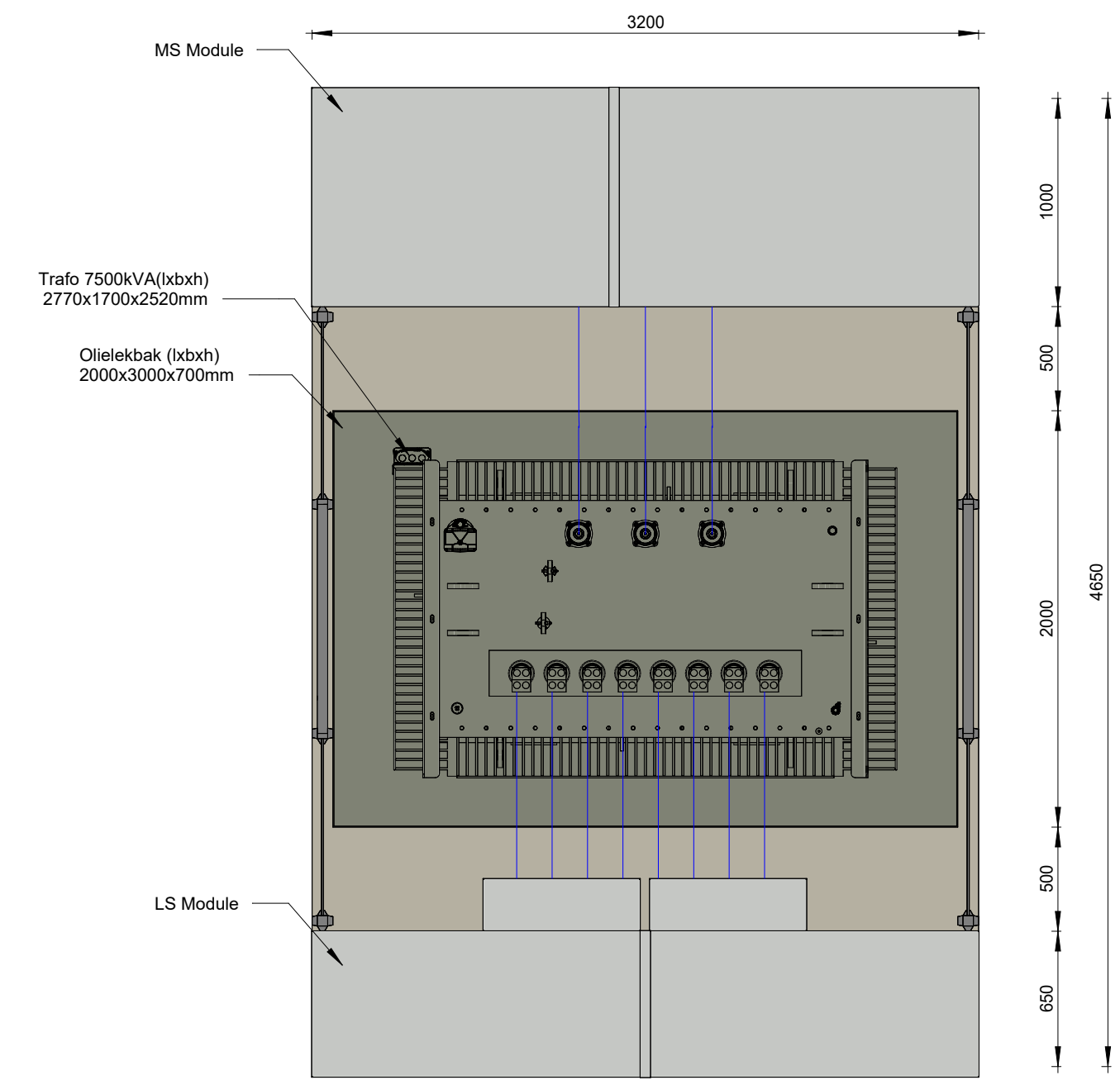
BOVENAANZICHT
