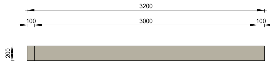
VLOERPLAAT RECHTERAANZICHT
