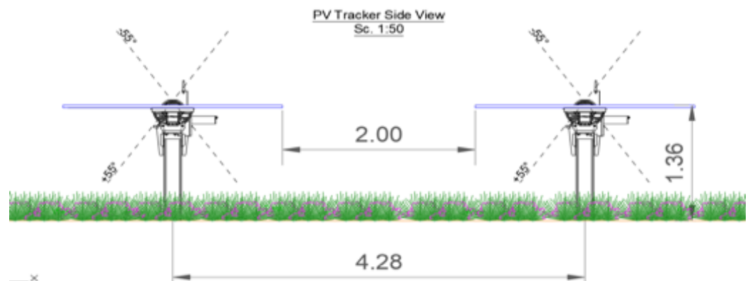
Voorbeeld doorsnede twee rijen zon-volgend park
