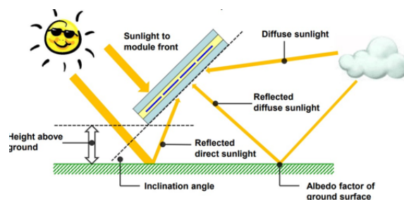
Bi-faciale panelen vangen licht aan beide kanten
