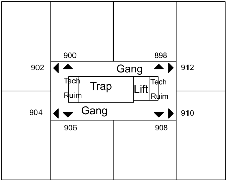
Blok 8 4e Verdieping
