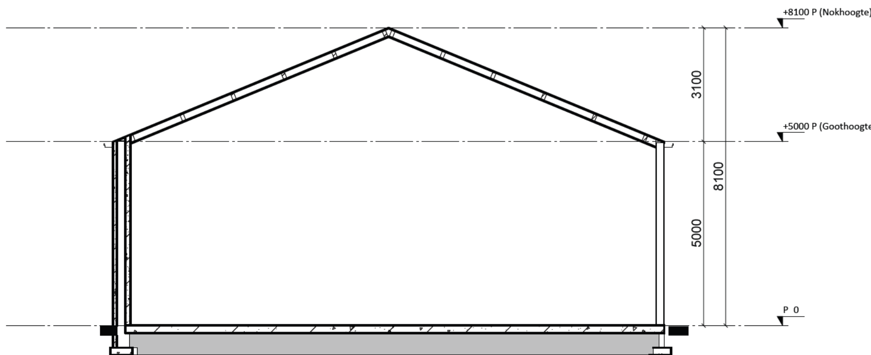
Doorsnede C' - C'
