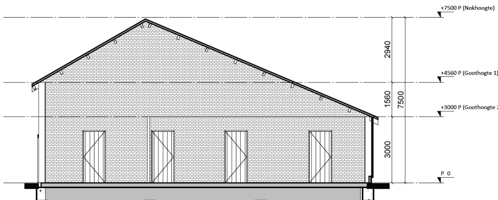
Doorsnede B' - B'
