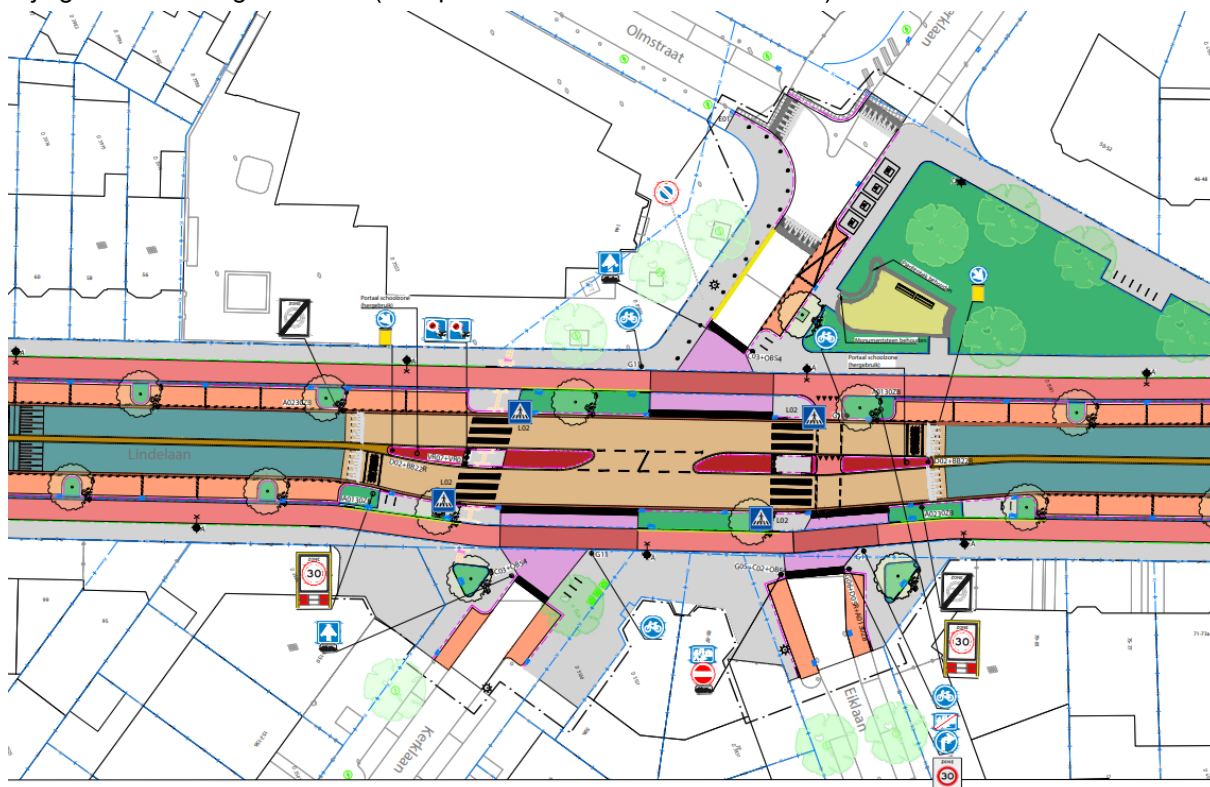
Bijlage 1 toekomstige 30-zone (kruispunt Lindelaan-Kerklaan-Eiklaan)
