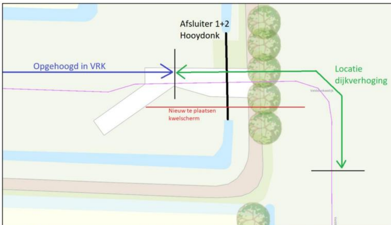
Figuur 1: Locatie dijkverhoging (voor exacte locatie kwelscherm raadpleeg het ontwerp document)
