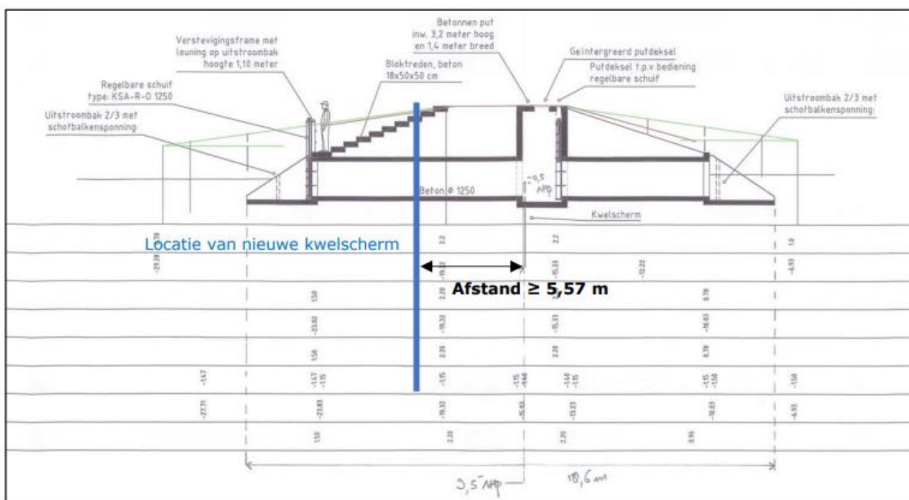
Figuur 2: Locatie nieuwe kwelscherm
