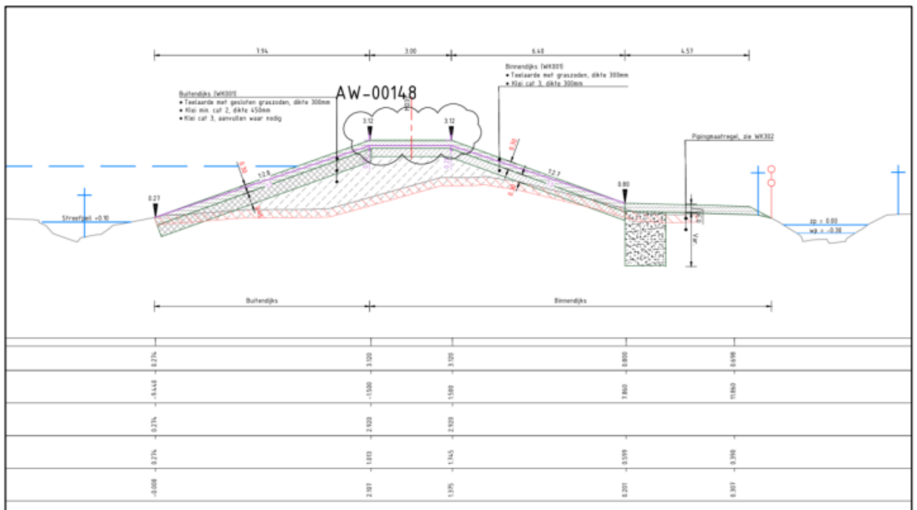
Figuur 3: Aanlegtekening dijkvak DP06-15
