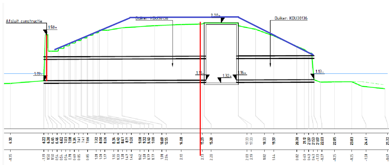
Figuur 1: Ophoging dwarsprofiel
