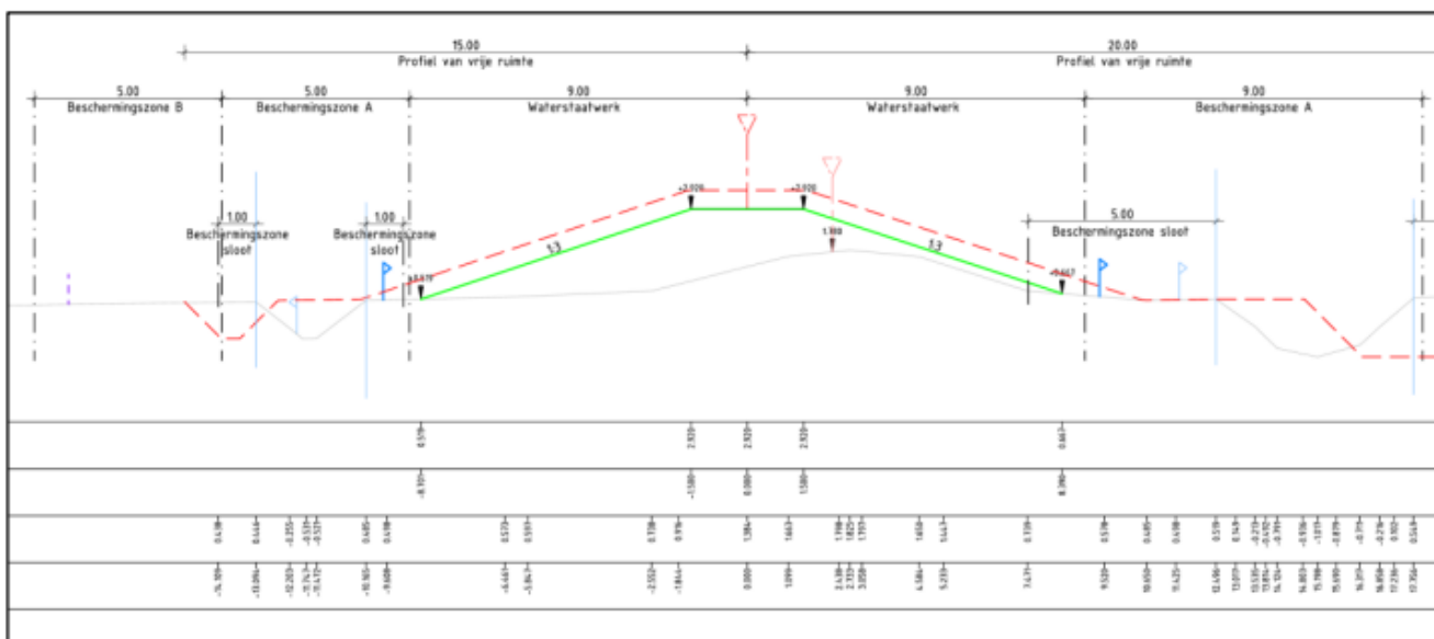
Figuur 2: Leggertekening dijkvak DP06-15
