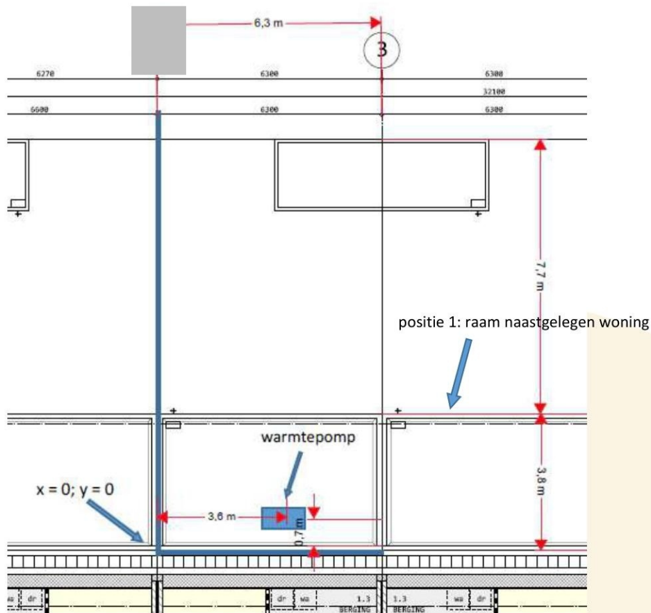
Figuur 2: geometrische uitgangspunten
